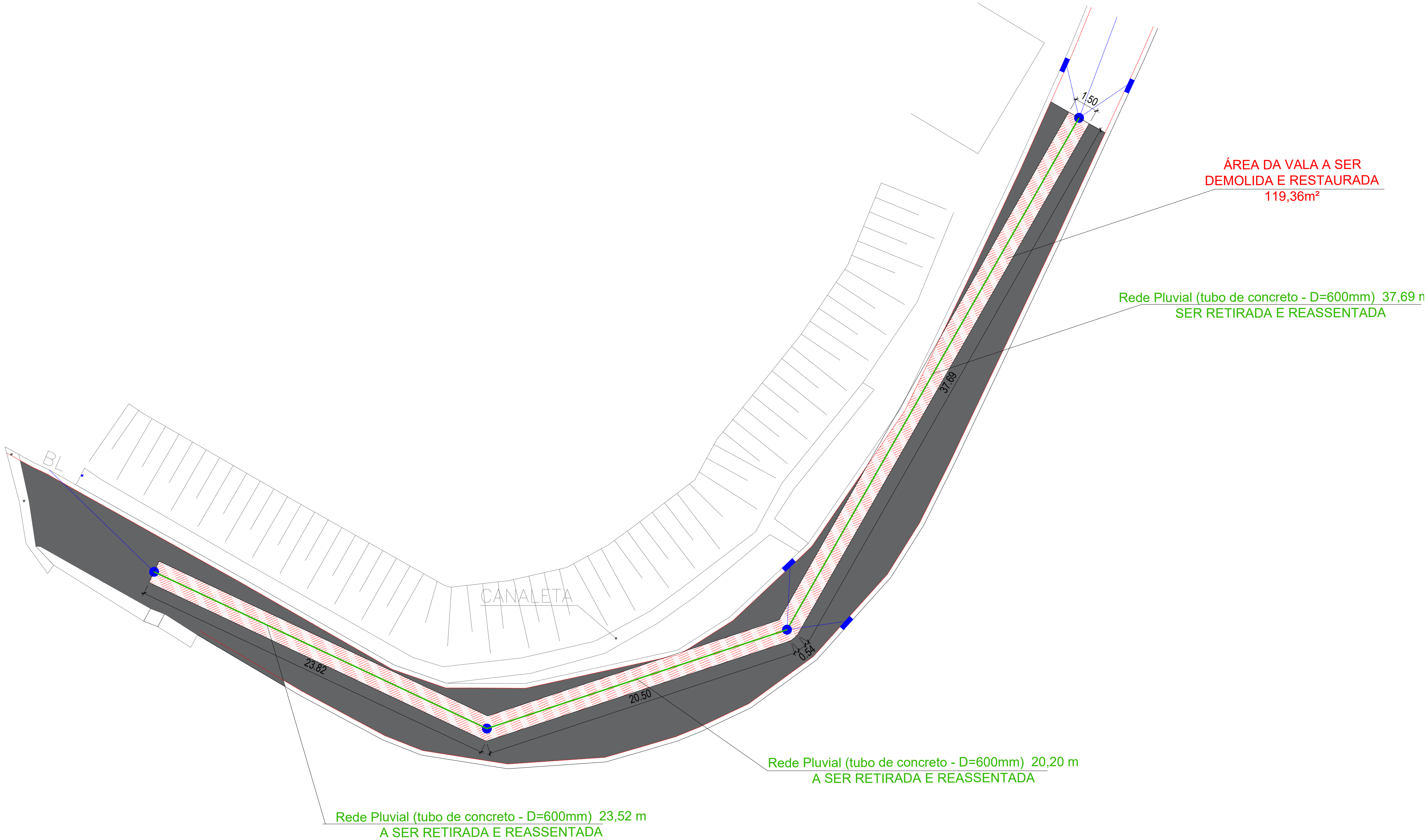
2 PROJETO DE DEMOLIÇÃO E REPADO ESCALA 1:150
