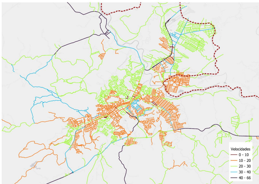
Figura 23 - Sistema Viário, destacando locais de retenção nos picos
