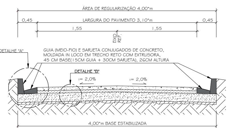
SEÇÃO TRANSVERSAL PAVIMENTO TIPO RUA MARIA AUGUSTA TIBÃES SEM ESCALA
