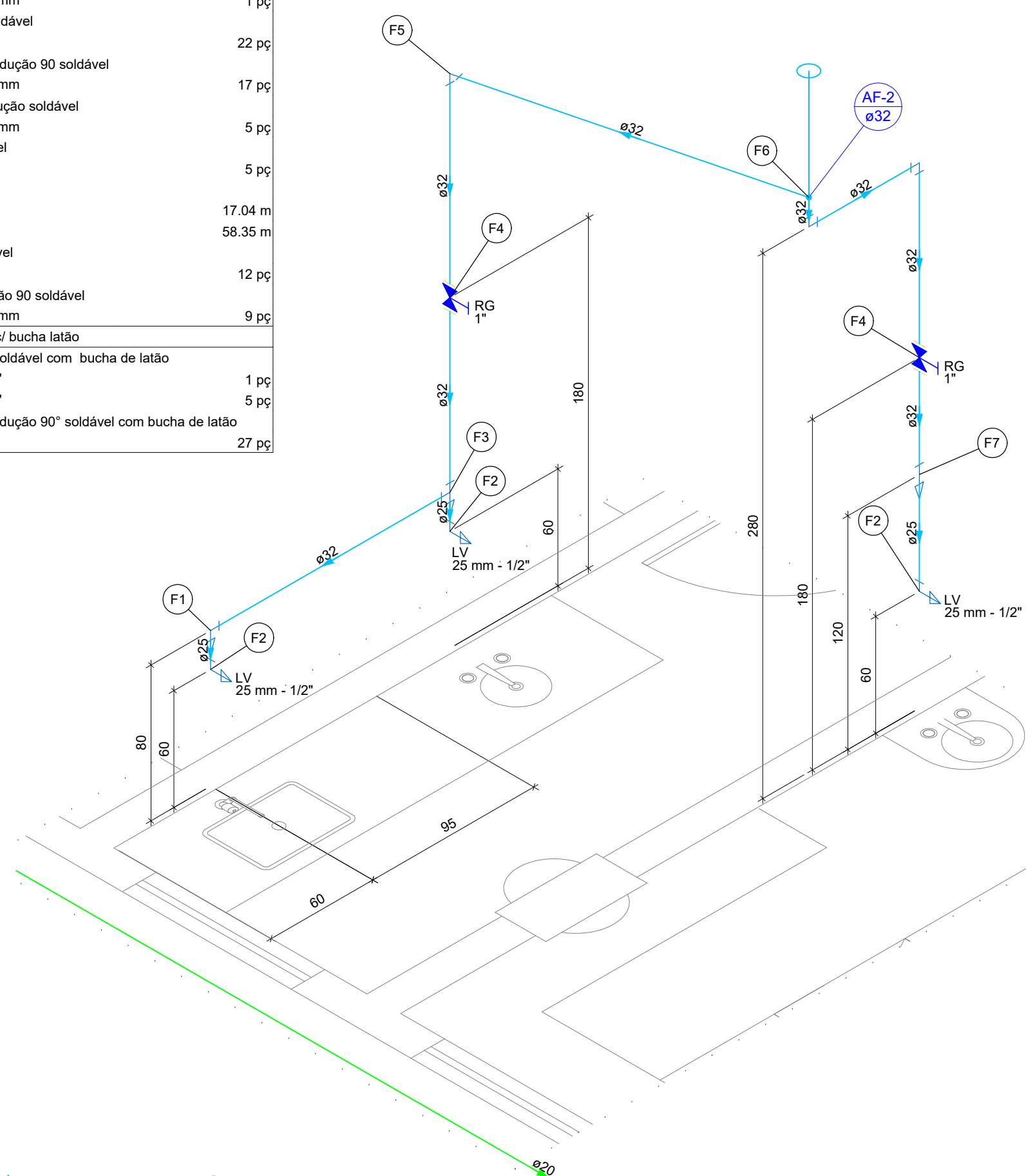
DETALHE HID-1
