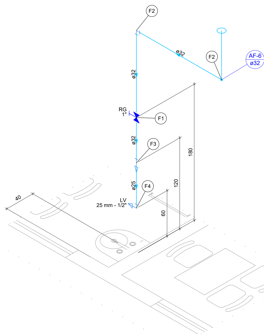
DETALHE HID-5
