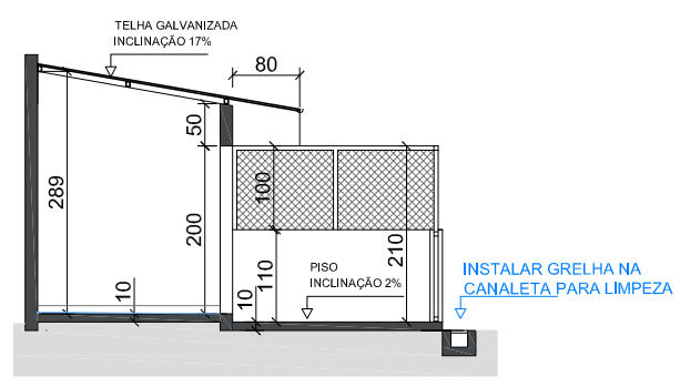
CORTE TRANSVERSAL esc. 1:100
