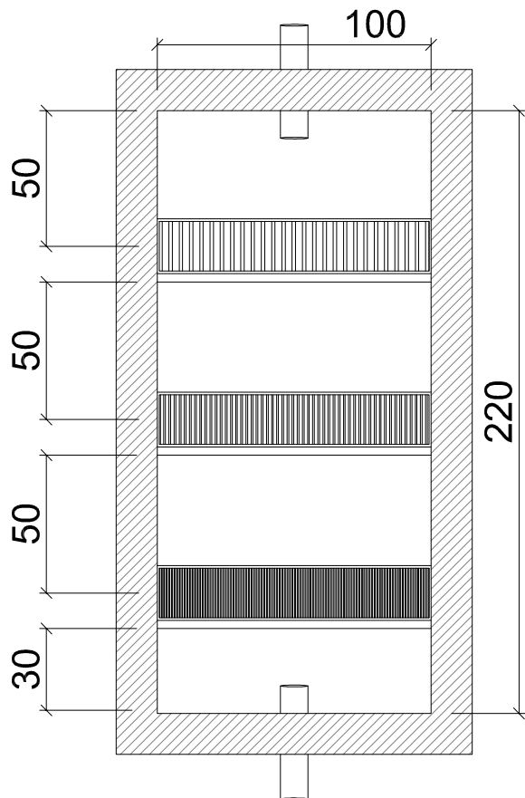
PLANTA BAIXA - CAIXA DE GRADEAMENTO esc. 1:25
