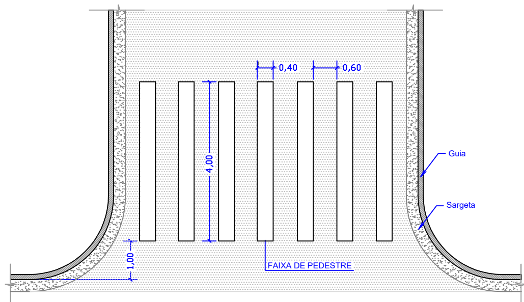
DETALHE DE FAIXA DE PEDESTRE ZEBRADA (F) (Escala 1:100)
