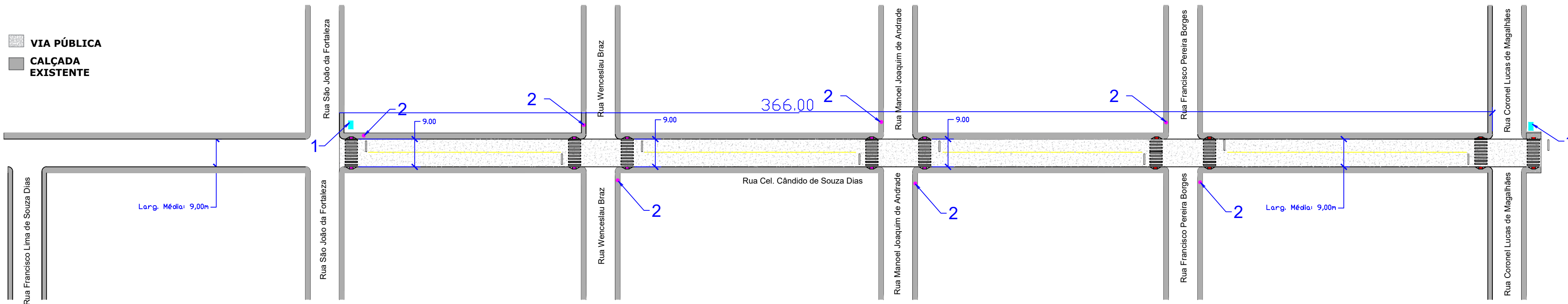
DETALHE DE SINALIZAÇÃO COMPLEMENTAR (DA/R) (Escala 1:50)
