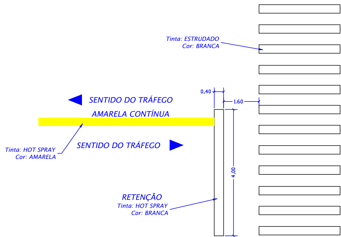
DETALHE DE SINALIZAÇÃO COMPLEMENTAR (DA/R) (Escala 1:50)
