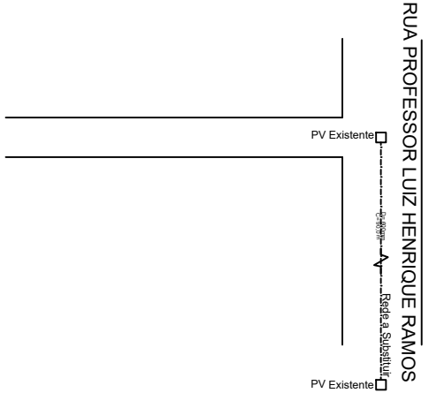
DRENAGEM RUA PROF. LUIZ HENRIQUE RAMOS SEM ESCALA
