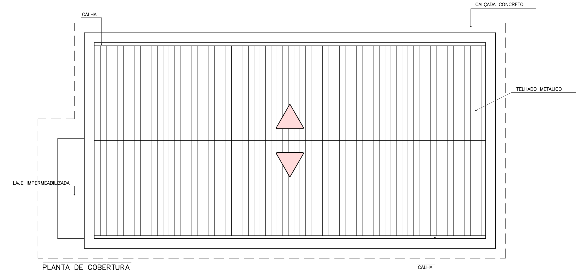
PLANTA DE COBERTURA ESC. 1:100
