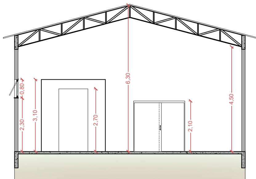
CORTE CC ESC. 1:100
