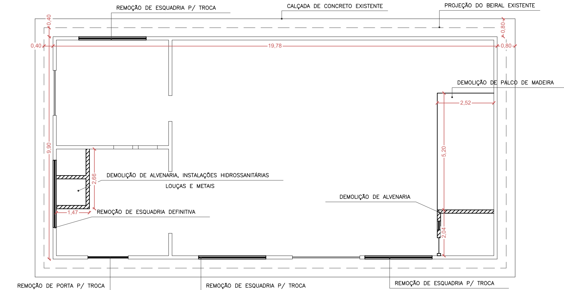
PLANTA BAIXA EXISTENTE NO LOCAL ESC. 1:100
