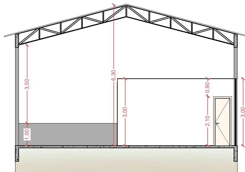
CORTE DD ESC. 1:100
