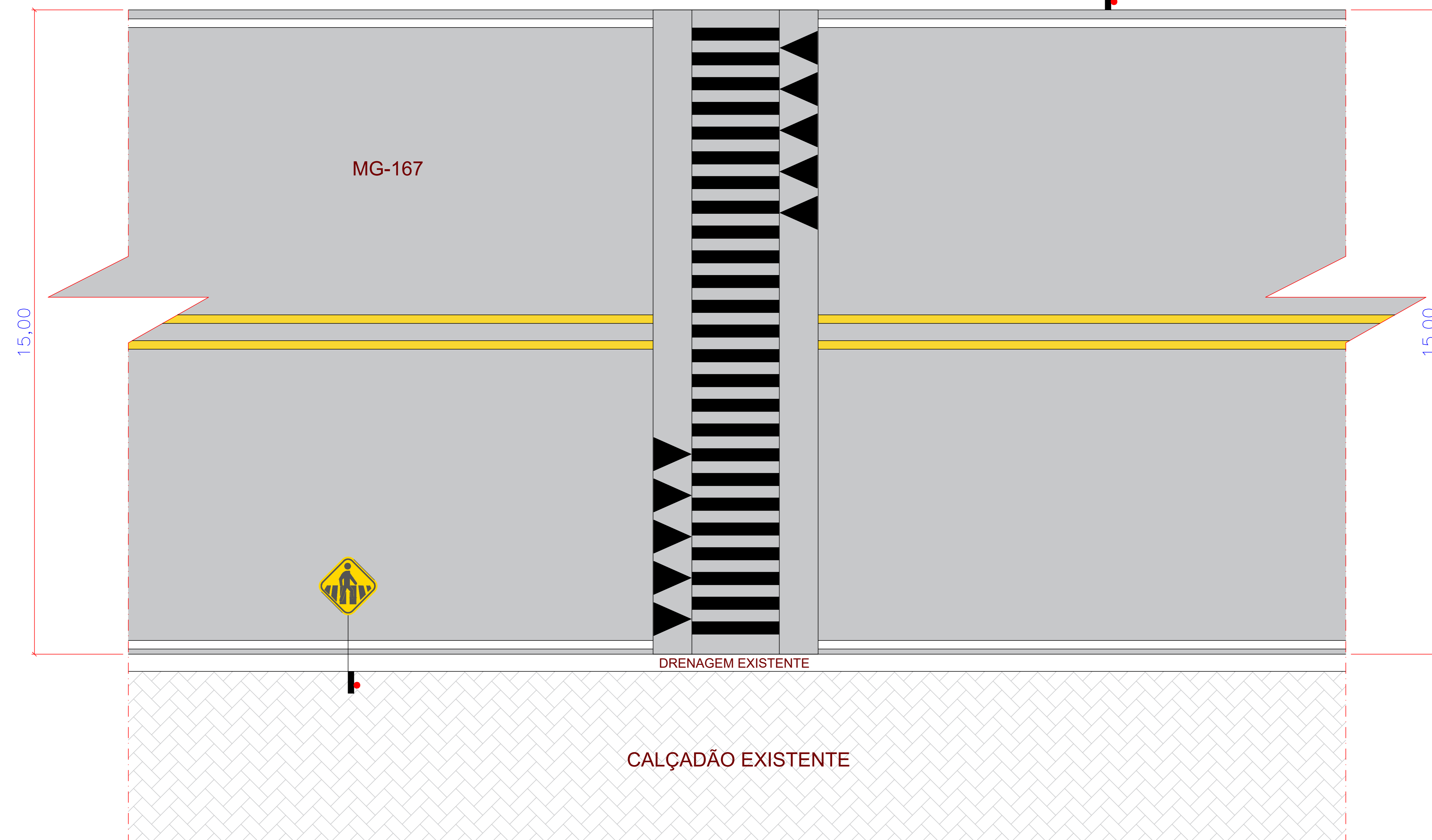
SINALIZAÇÃO HORIZONTAL BR-167 Escala 1:100
