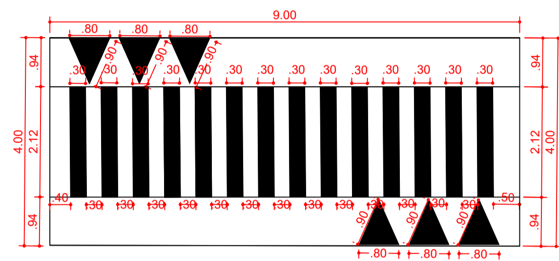
SINALIZAÇÃO HORIZONTAL TRAVESSIA ELEVADA BR-167 Escala 1:100
