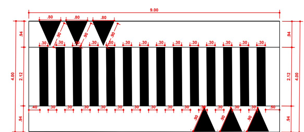
SINALIZAÇÃO HORIZONTAL TRAVESSIA ELEVADA BR-167 Escala: 1:100
