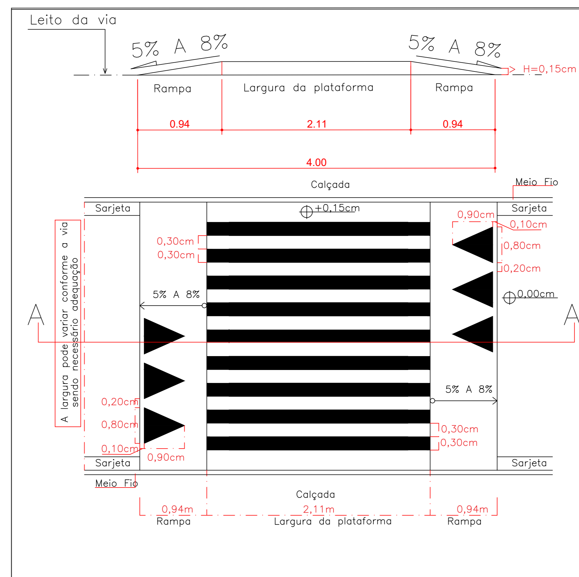
Medidas sinalização horizontal Escala 1:250
