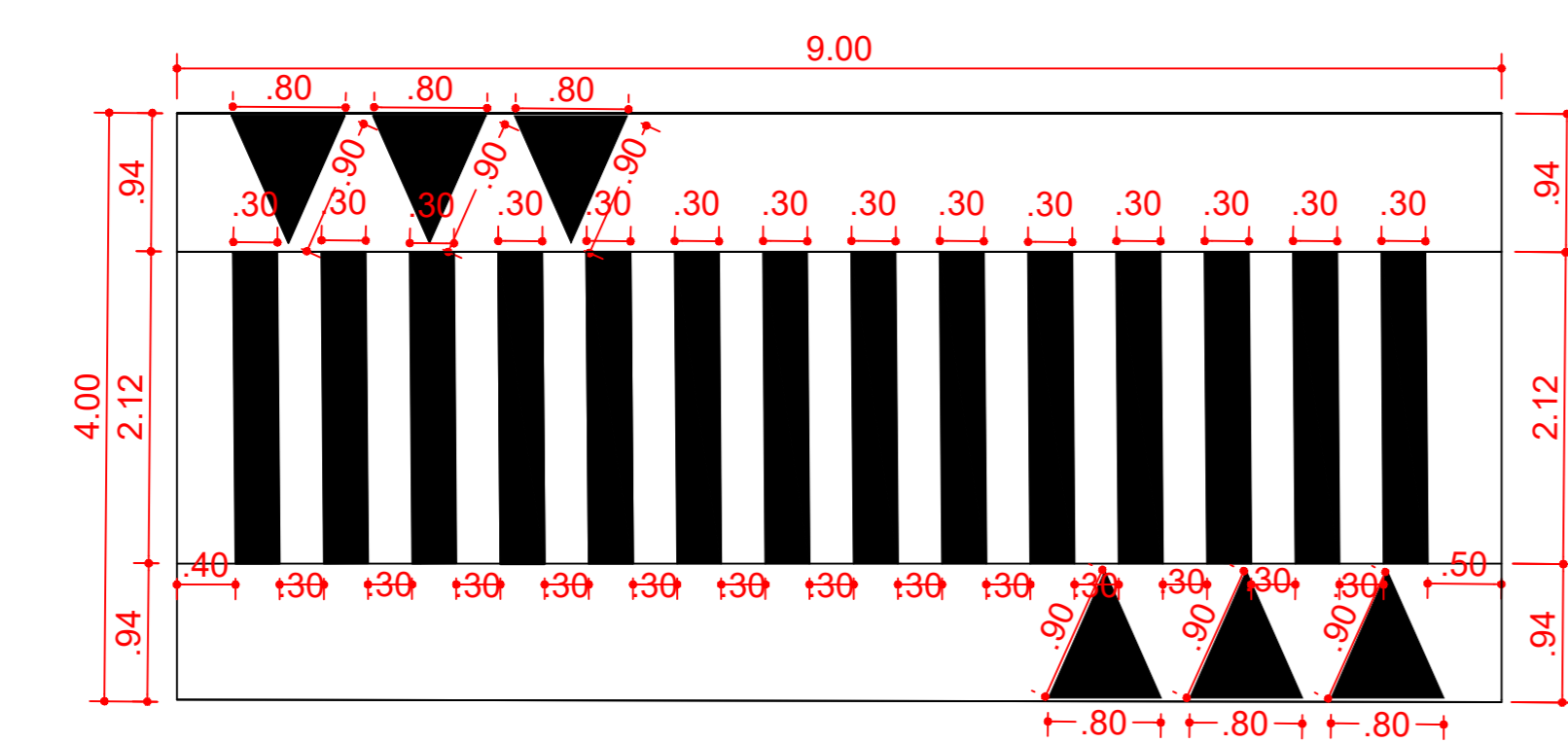
SINALIZAÇÃO HORIZONTAL TRAVESSIA ELEVADA BR-167 Escala 1:100
