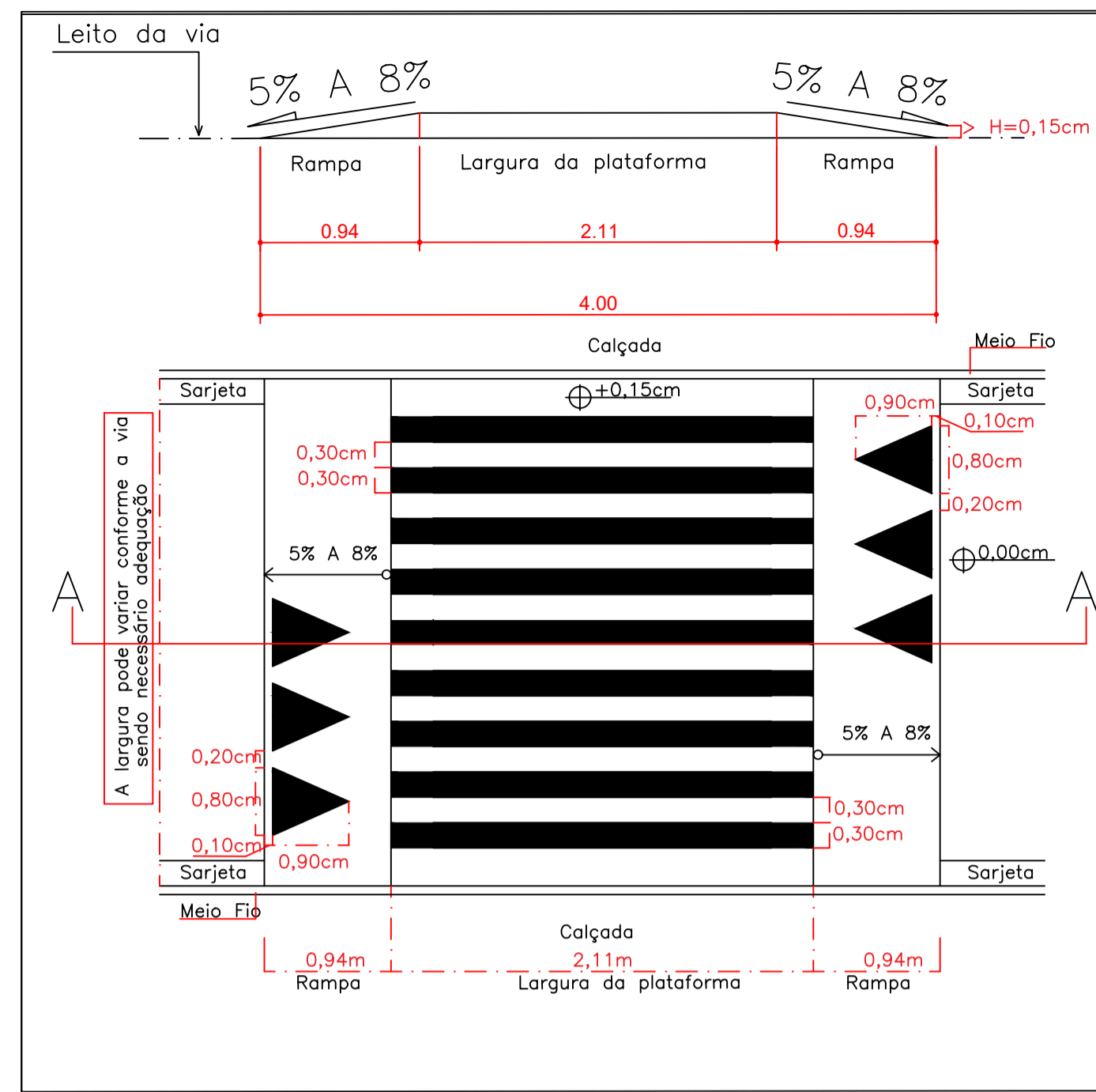
Medidas sinalização horizontal Escala 1:250
