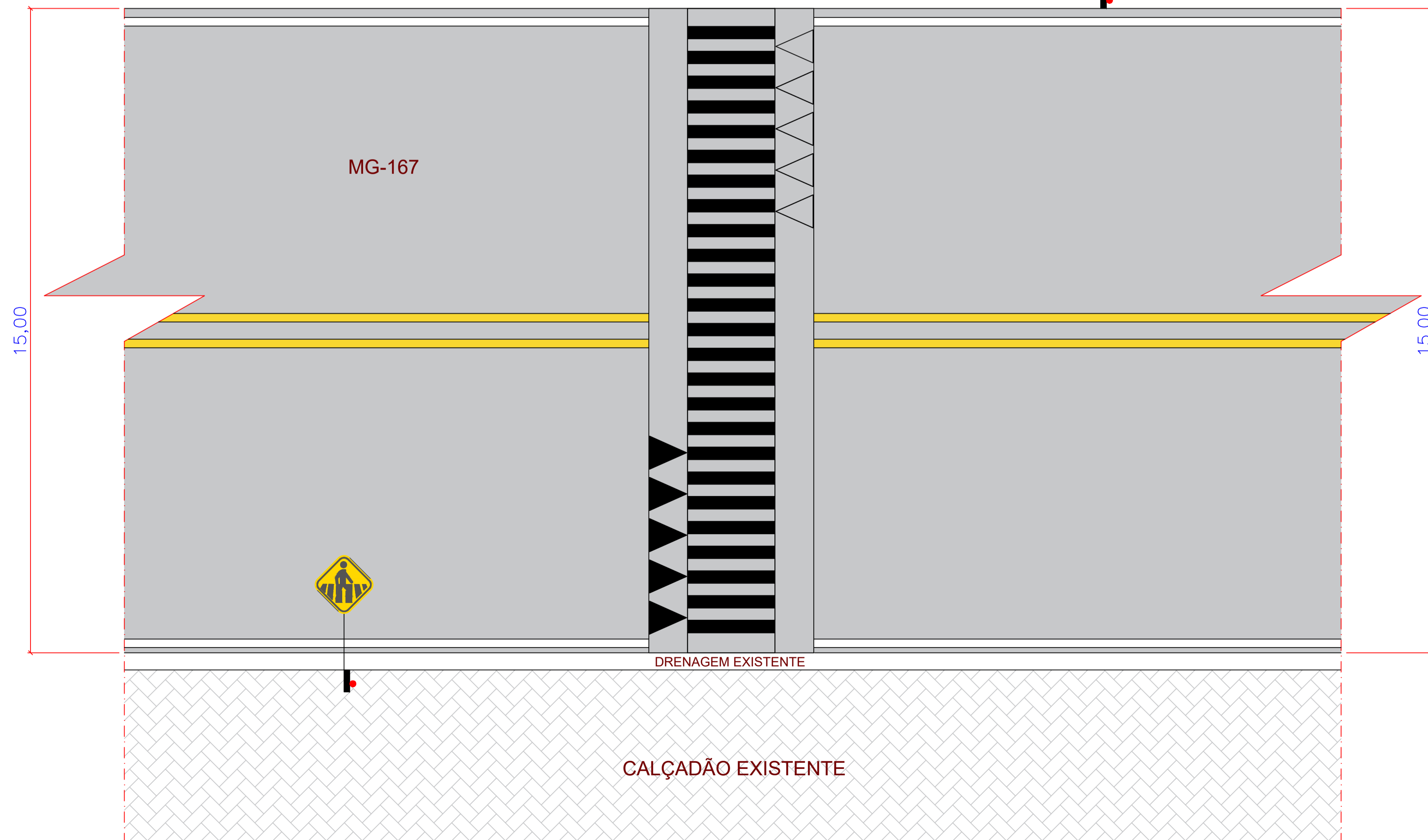
SINALIZAÇÃO HORIZONTAL BR-167 Escala 1:100
