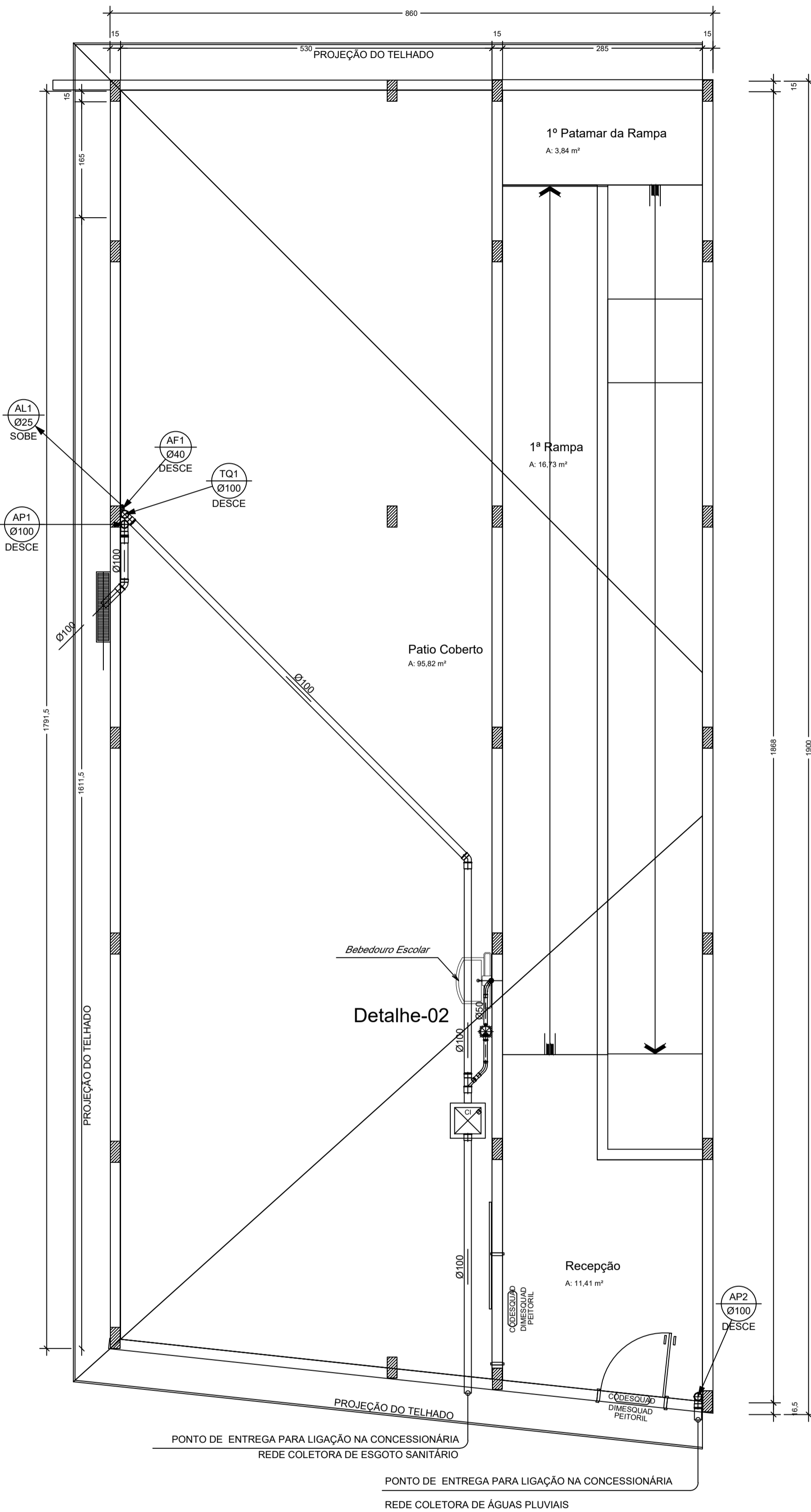
Planta Baixa Sistema Hidrossanitário
