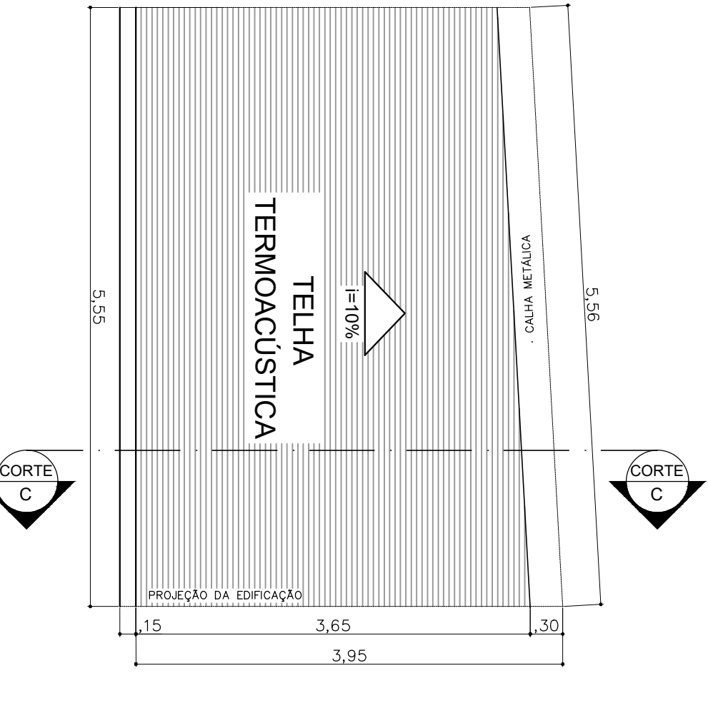
PLANTA DE COBERTURA ÁREA DE SERVIÇO Esc. 1:50
