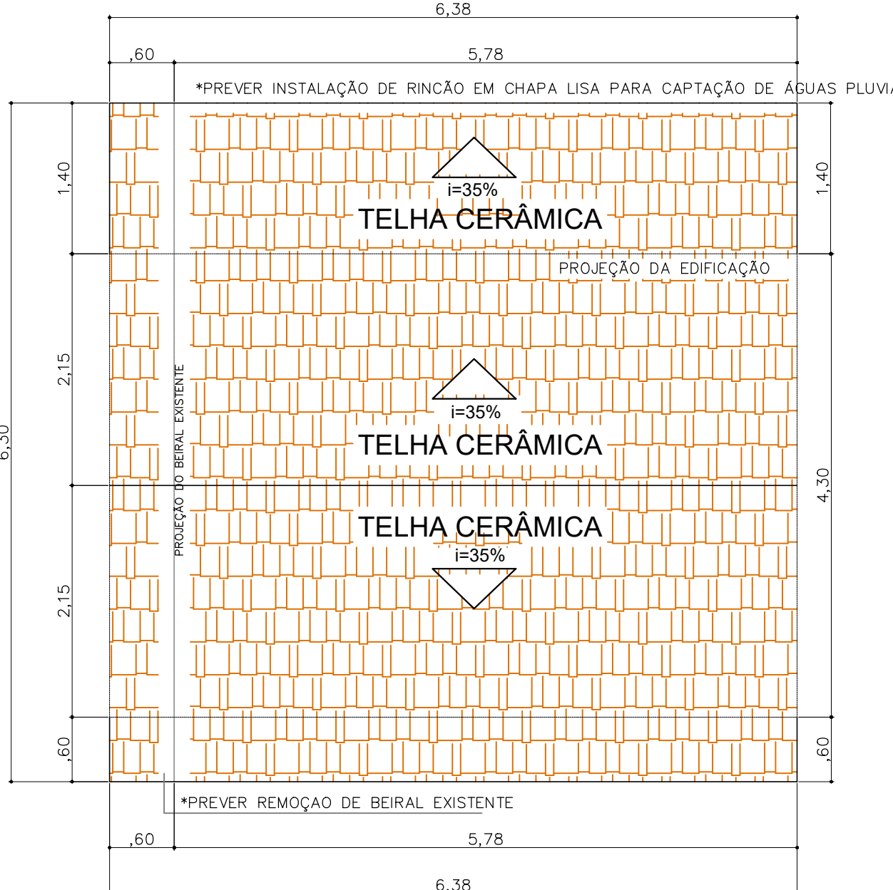
PLANTA DE COBERTURA SALA DE RECREAÇÃO Esc. 1:50
