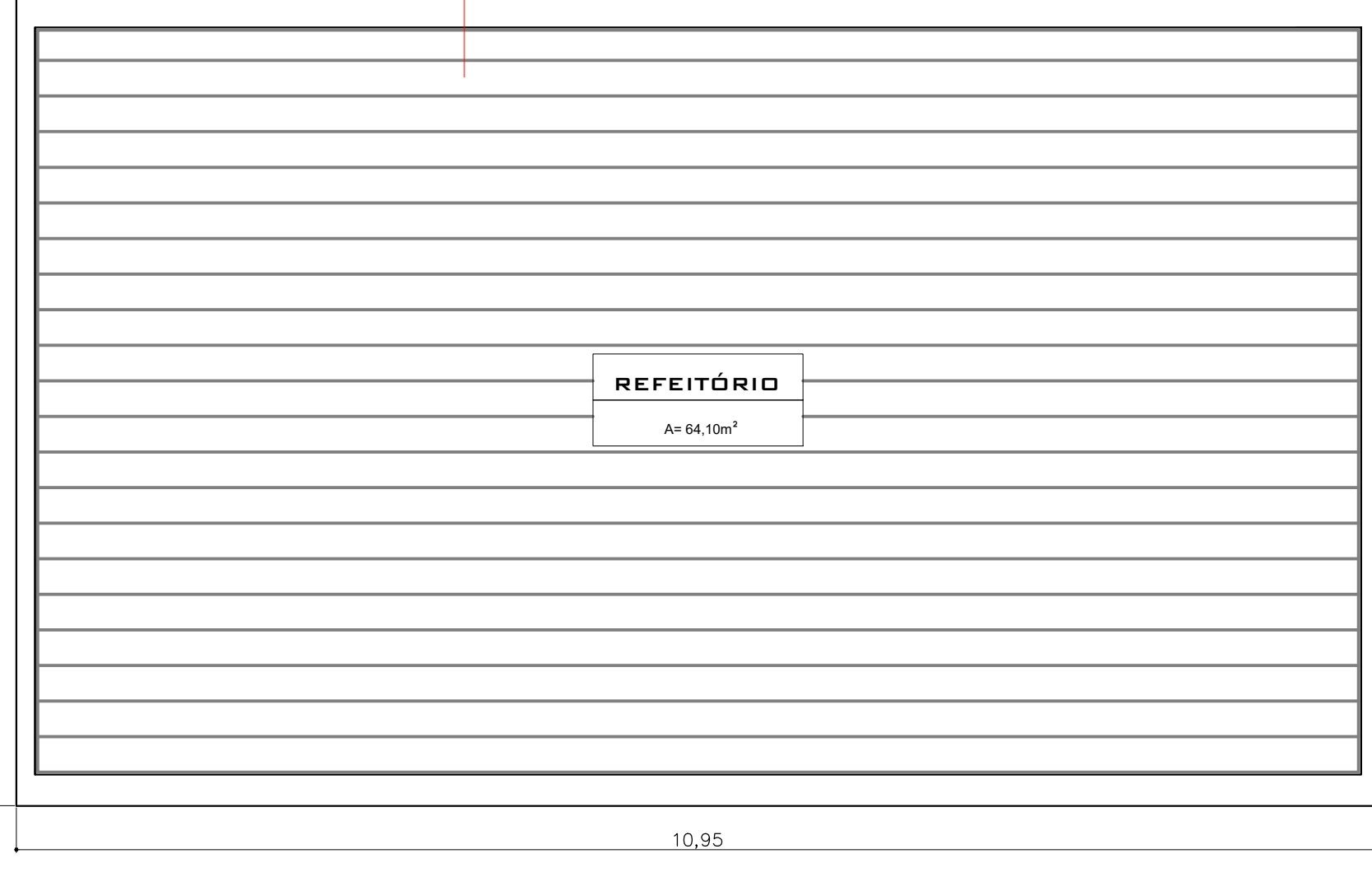
PLANTA DE FORRO REFEITÓRIO Esc. 1:50
