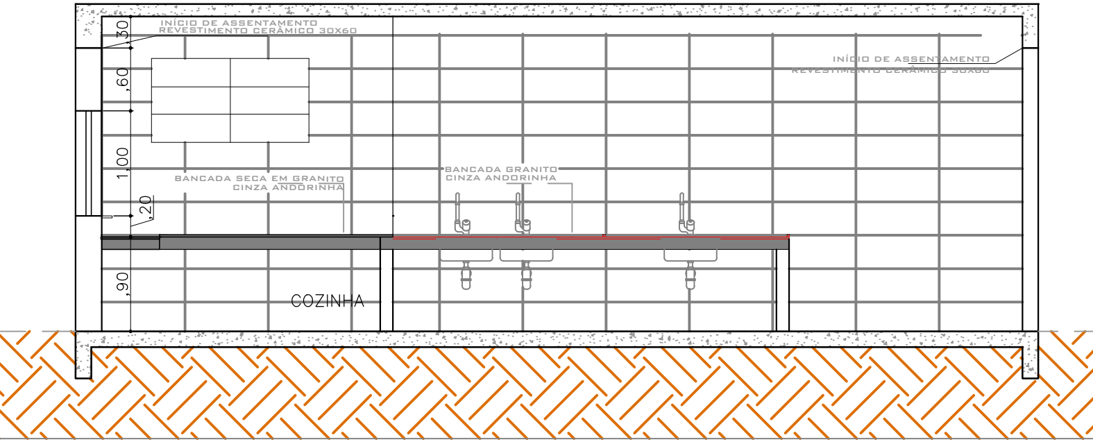
ELEVACÃO A Esc. 1:50
