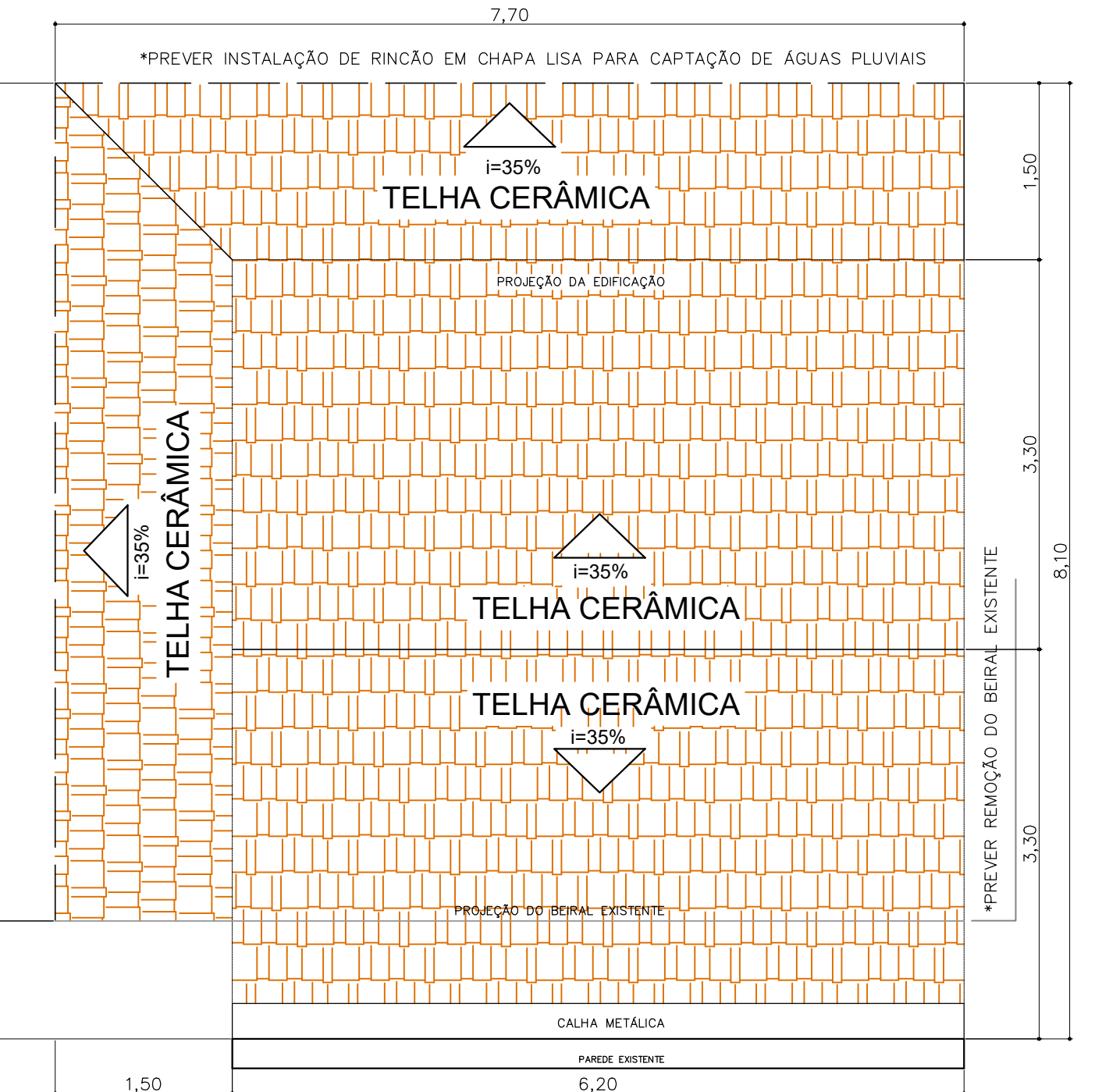
PLANTA DE COBERTURA SALA DE AULA (AMPLIAÇÃO) Esc. 1:50
