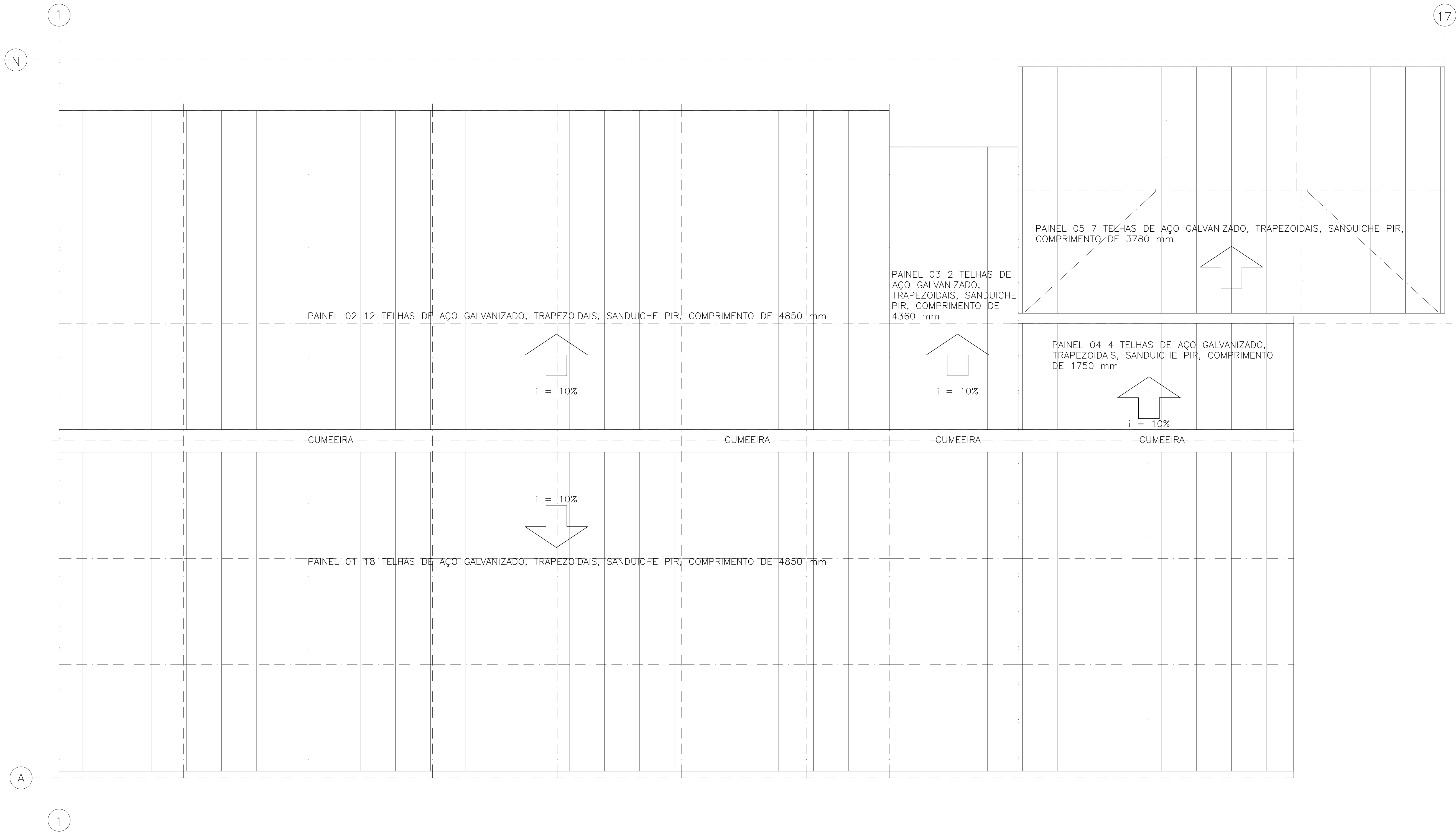
PLANO DE TELHAS DA COBERTURA
