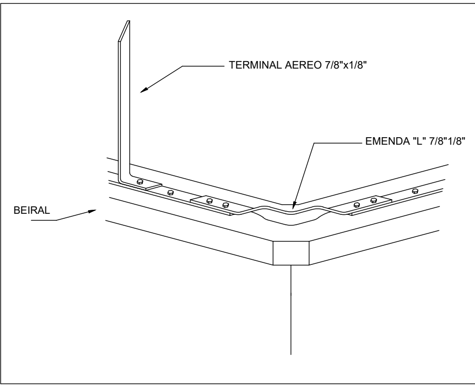
FIXAÇÃO BARRA CHATA SEM ESCALA
