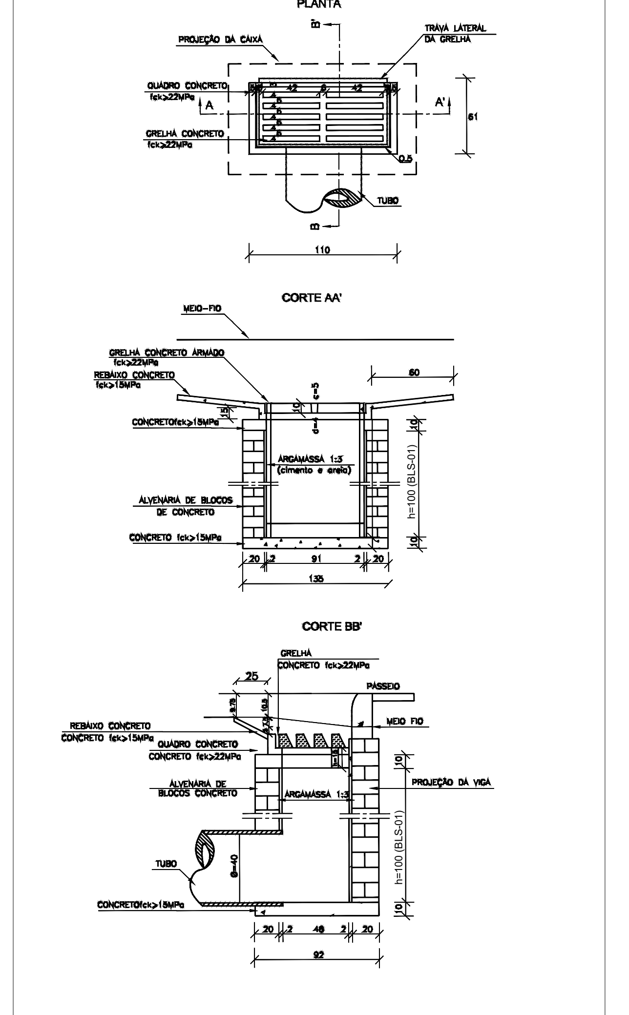
BOCA DE LOBO SIMPLES COM GRELHA DE CONCRETO TIPO BLS 01
