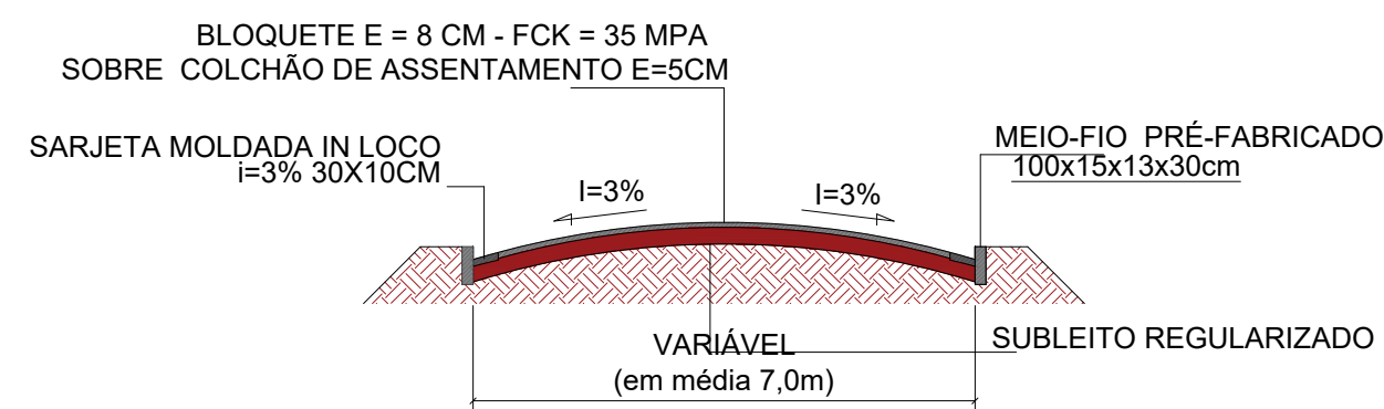
SEÇÃO TRANSVERSAL TIPO COM SARJETA DOS DOIS LADOS ESCALA 1/100
