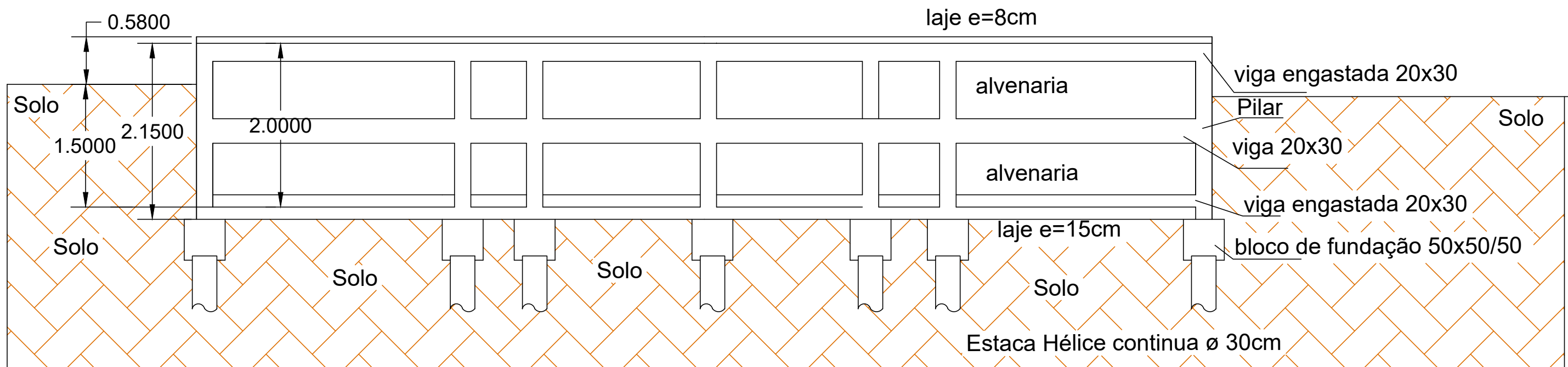
CORTE AA
