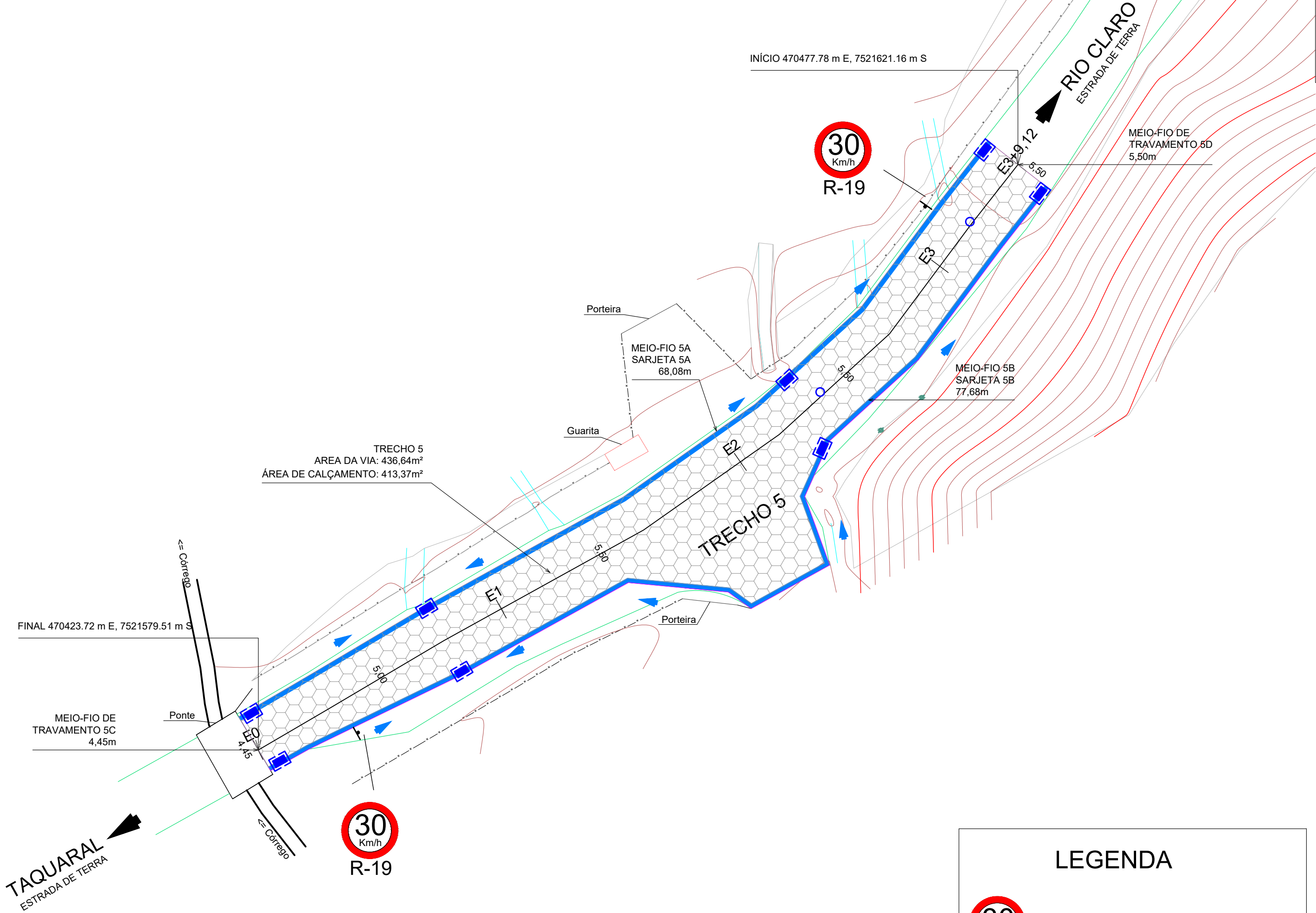
BAIRRO RIO CLARO - TRECHO 05 PLANTA DE CALÇAMENTO COM SINALIZAÇÃO ESCALA 1/250
