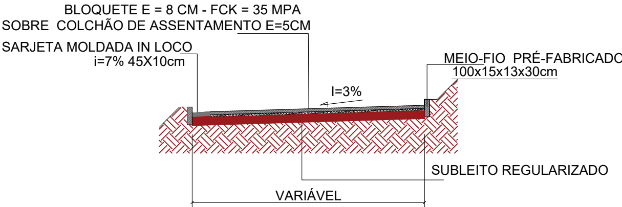
SEÇÃO TRANSVERSAL TIPO COM SARJETA APENAS DE UM LADO
