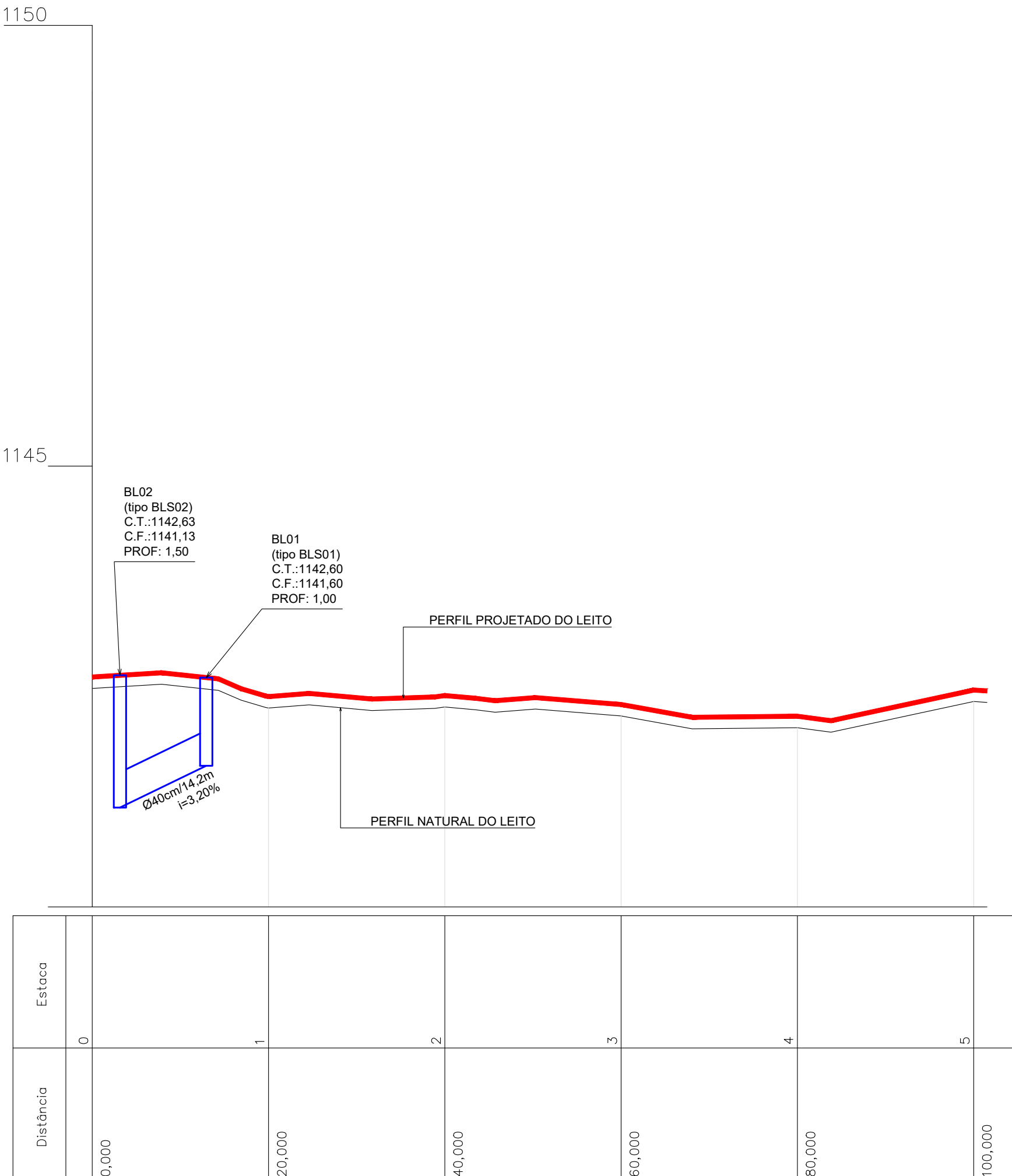
PERFIL LONGITUDINAL BAIRRO MORANGAL - TRECHO 04
