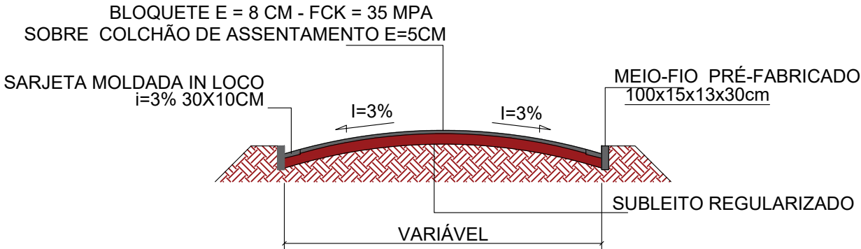
SEÇÃO TRANSVERSAL TIPO COM SARJETA DOS DOIS LADOS ESCALA 1/100
