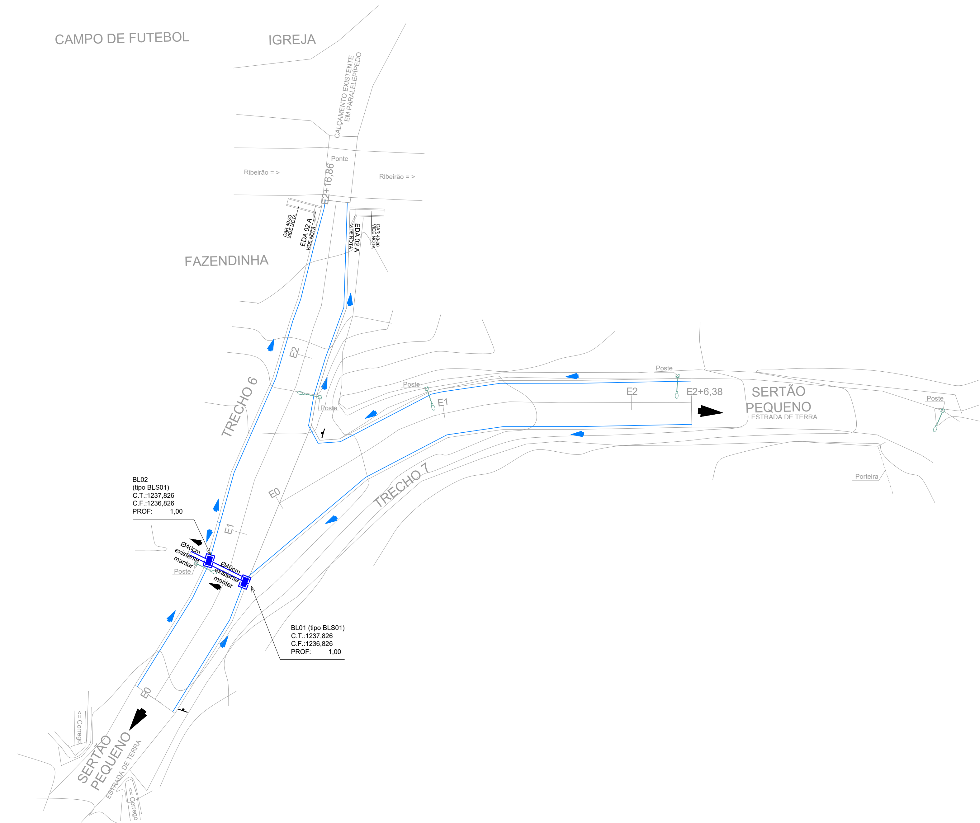
BAIRRO SERTÃO DE BAIXO (FAZENDINHA) - TRECHOS 06 E 07 PLANTA DE DRENAGEM ESCALA 1/250
