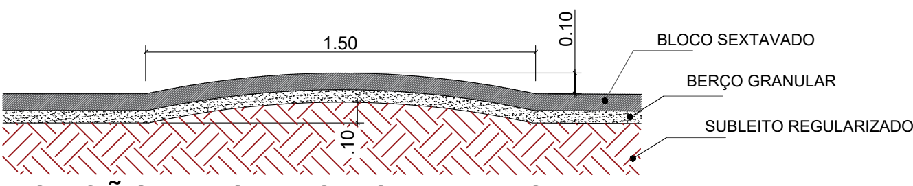
SEÇÃO-TIPO DAS LOMBADAS ESCALA 1/25
