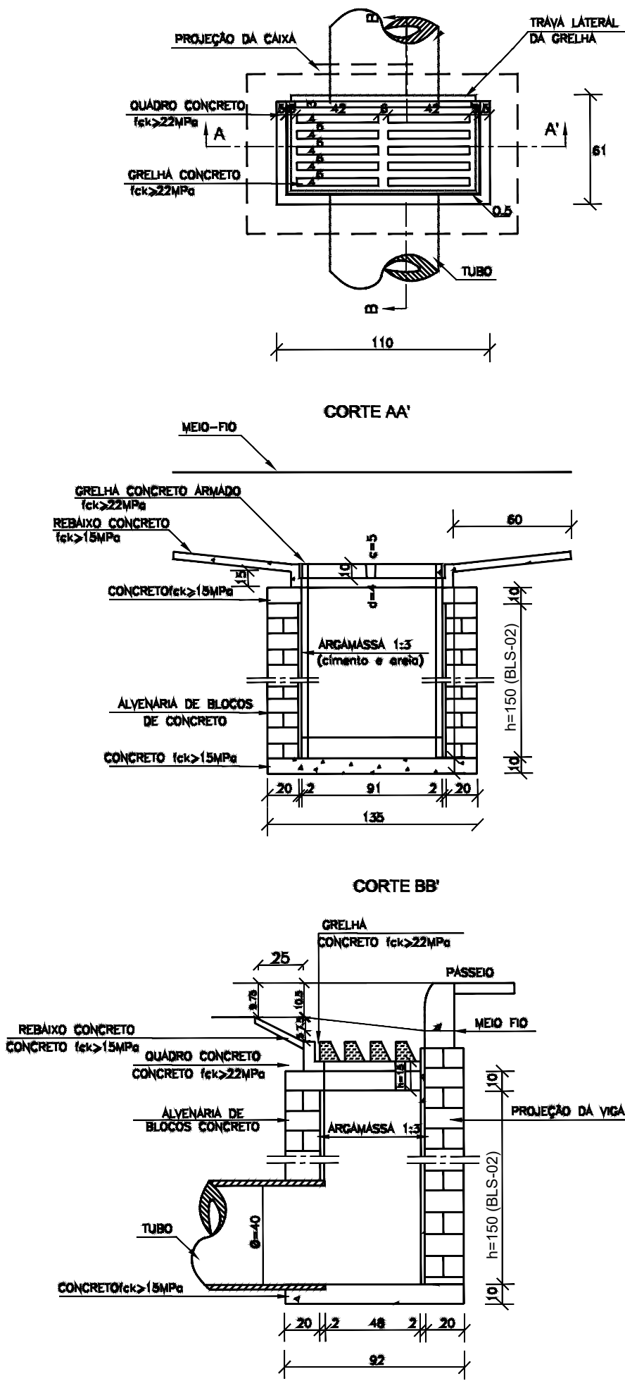
BL02 BOCA DE LOBO SIMPLES COM GRELHA DE CONCRETO TIPO BLS 02
