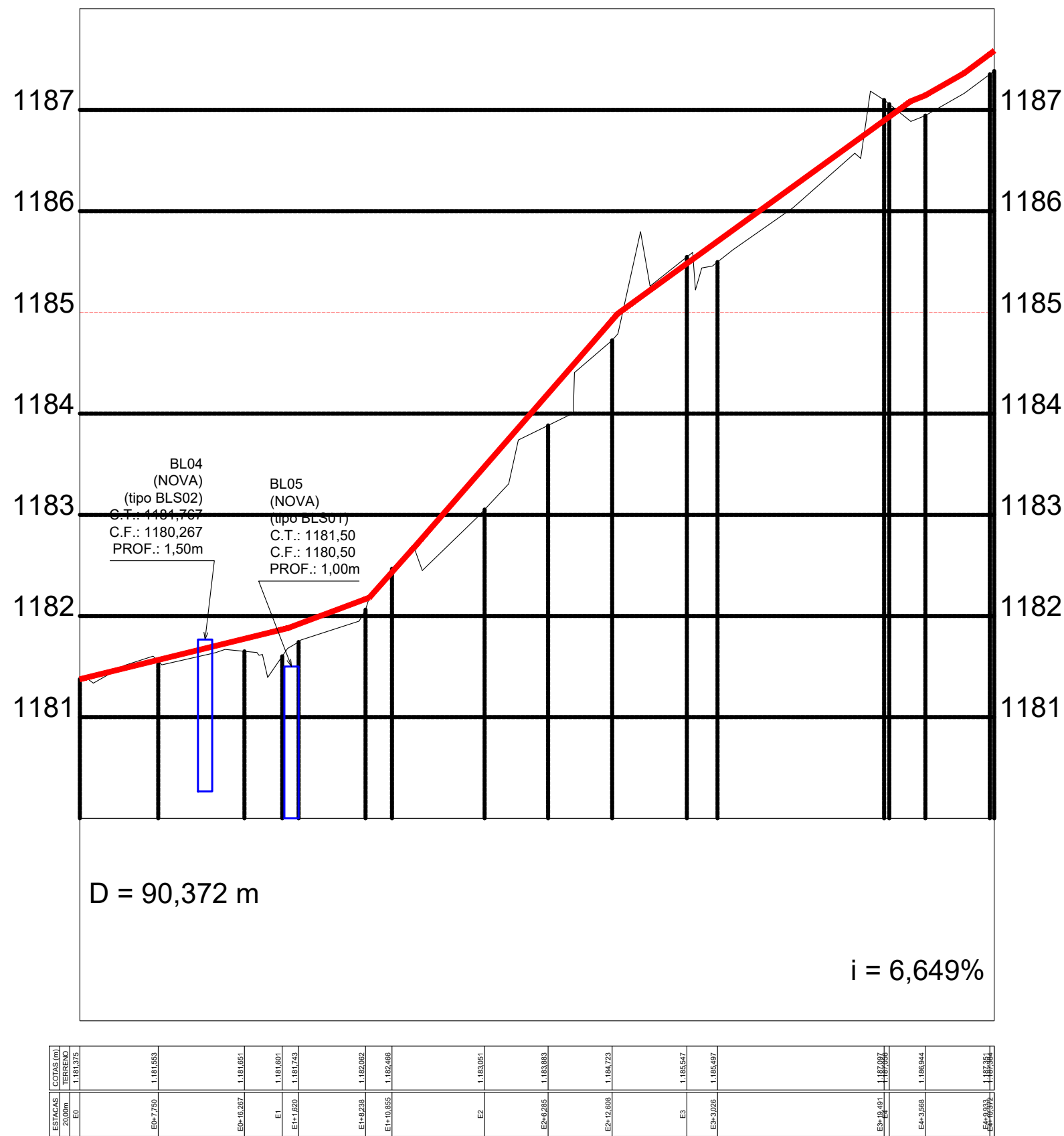
PERFIL LONGITUDINAL BAIRRO MONTEIRO - TRECHO 10 ESCALA HORIZONTAL 1/500 ESCALA VERTICAL 1/50
