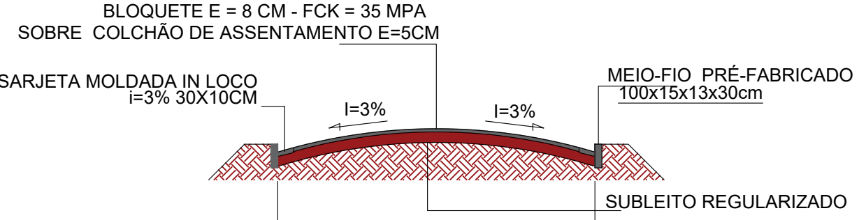
SEÇÃO TRANSVERSAL TIPO COM SARJETA DOS DOIS LADOS ESCALA 1/100
