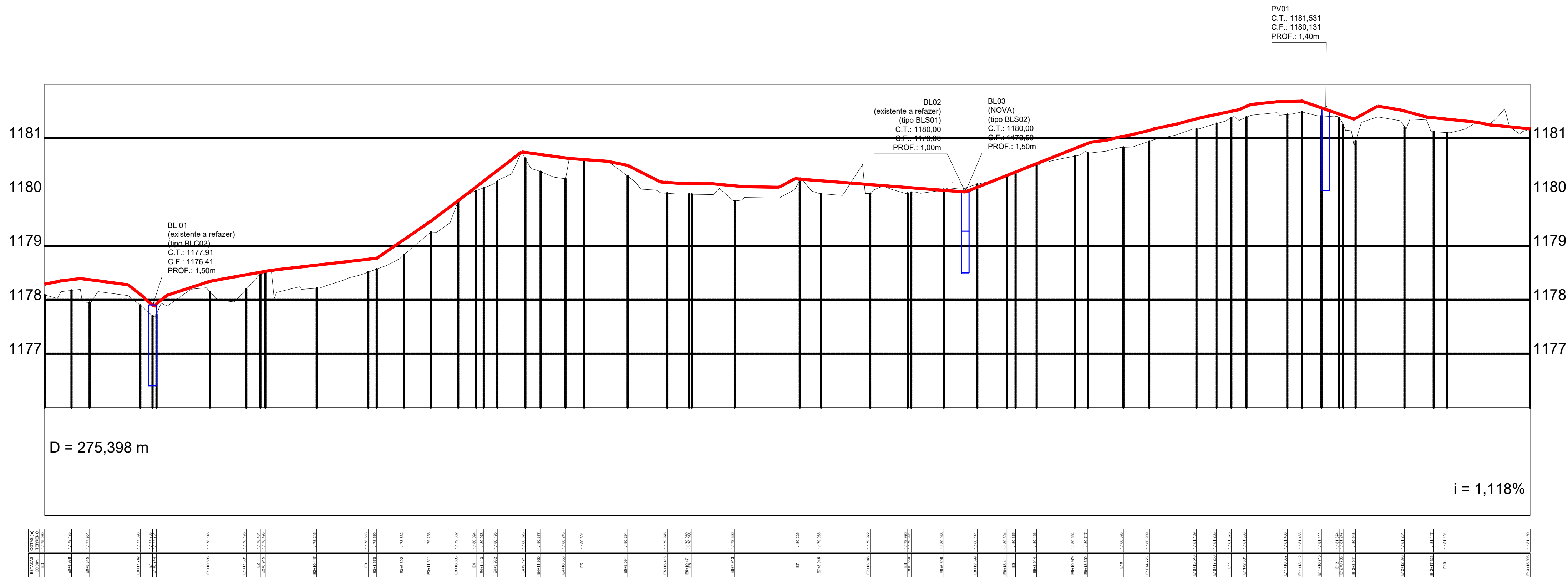
PERFIL LONGITUDINAL BAIRRO MONTEIRO - TRECHO 9 ESCALA HORIZONTAL 1/500 ESCALA VERTICAL 1/50
