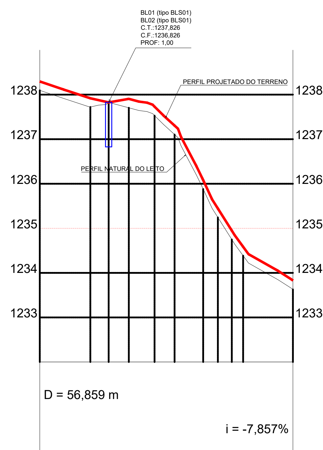
PERFIL LONGITUDINAL BAIRRO SERTÃO DE BAIXO (FAZENDINHA) - TRECHO 06 ESCALA HORIZONTAL 1/500 ESCALA VERTICAL 1/50
