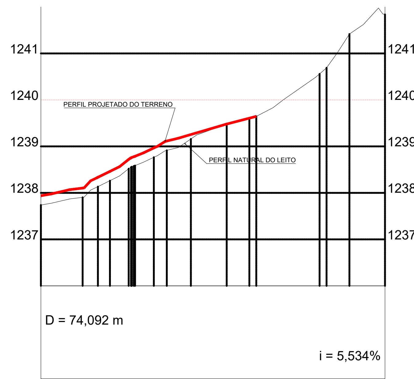
PERFIL LONGITUDINAL BAIRRO SERTÃO DE BAIXO (FAZENDINHA) - TRECHO 07 ESCALA HORIZONTAL 1/500 ESCALA VERTICAL 1/50
