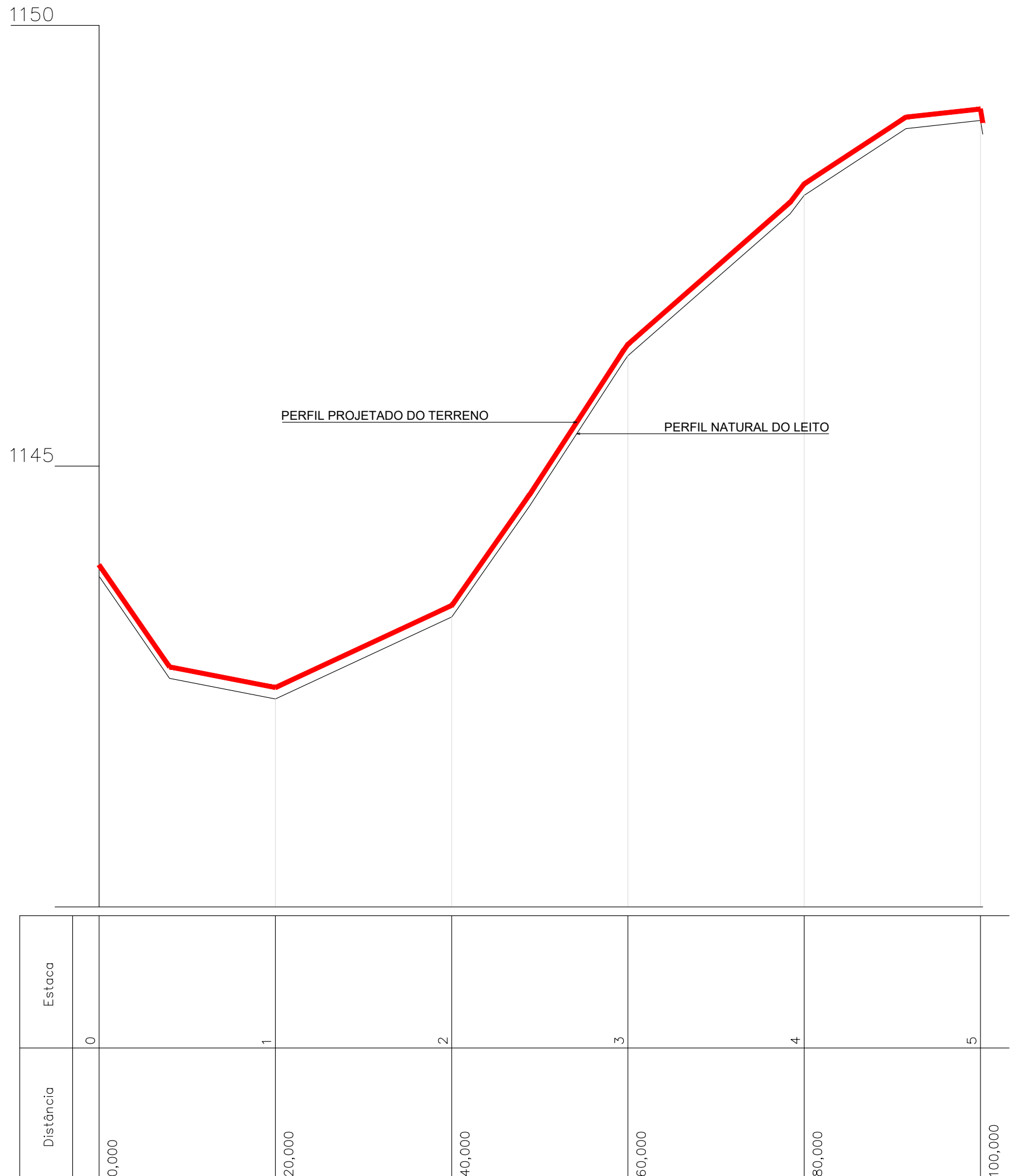
PERFIL LONGITUDINAL BAIRRO MORANGAL - TRECHO 03
