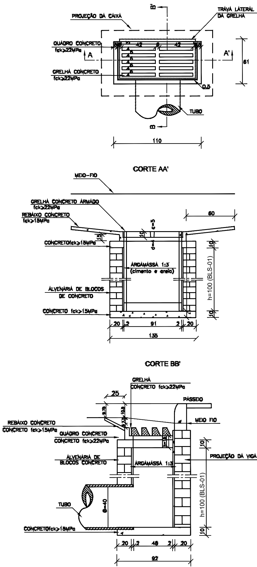
BL01 BOCA DE LOBO SIMPLES COM GRELHA DE CONCRETO TIPO BLS 01
