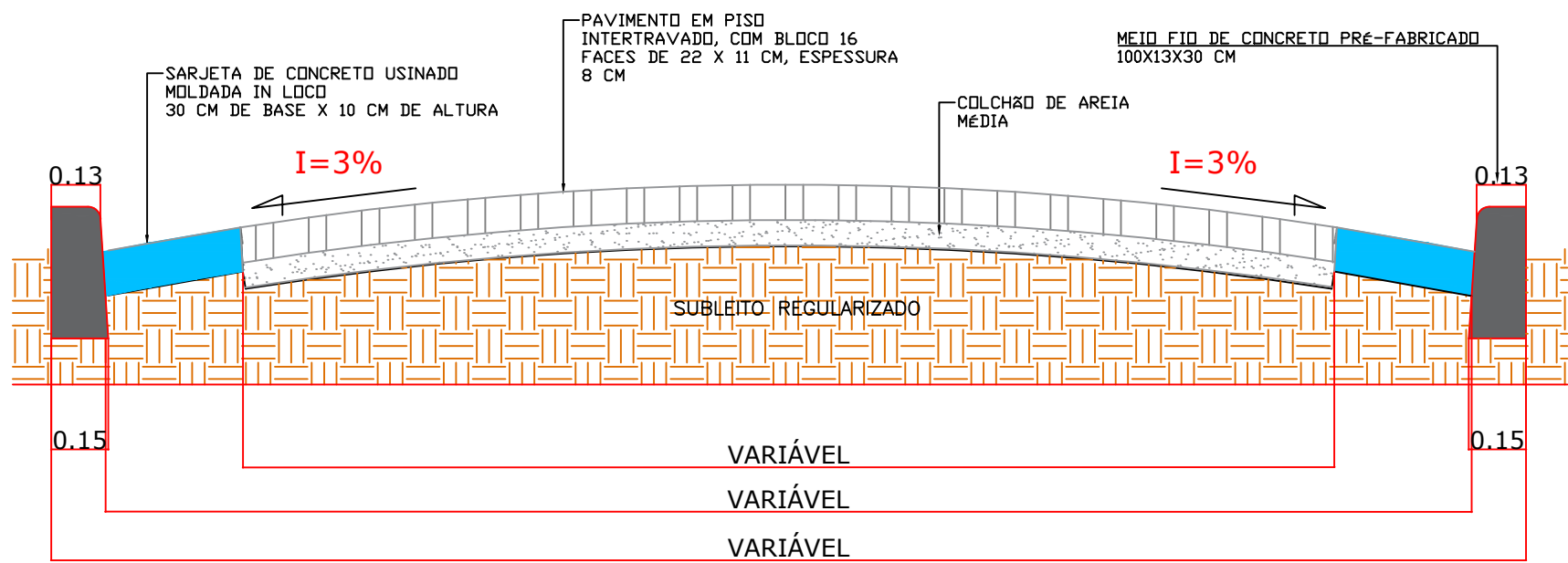
SESSÃO TRANSVERSAL PARA PAVIMENTAÇÃO EM PISO INTERTRAVADO SEM ESCALA
