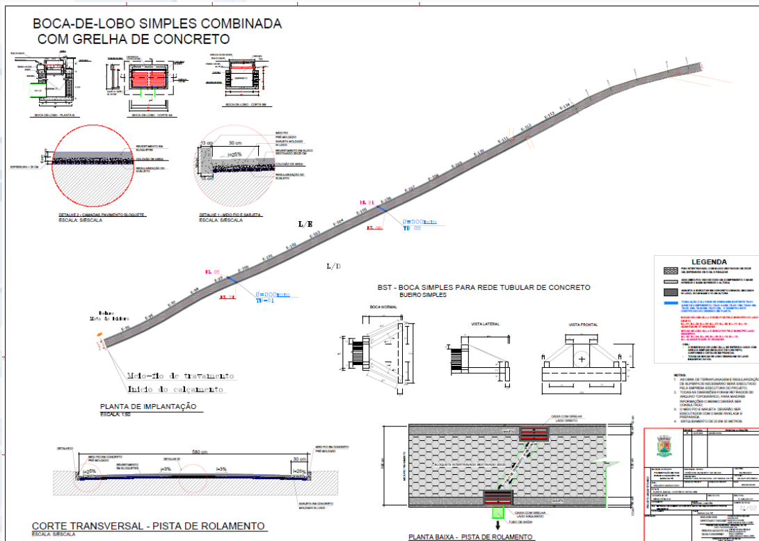
Figura 01 – Projeto de implantação do calçamento
