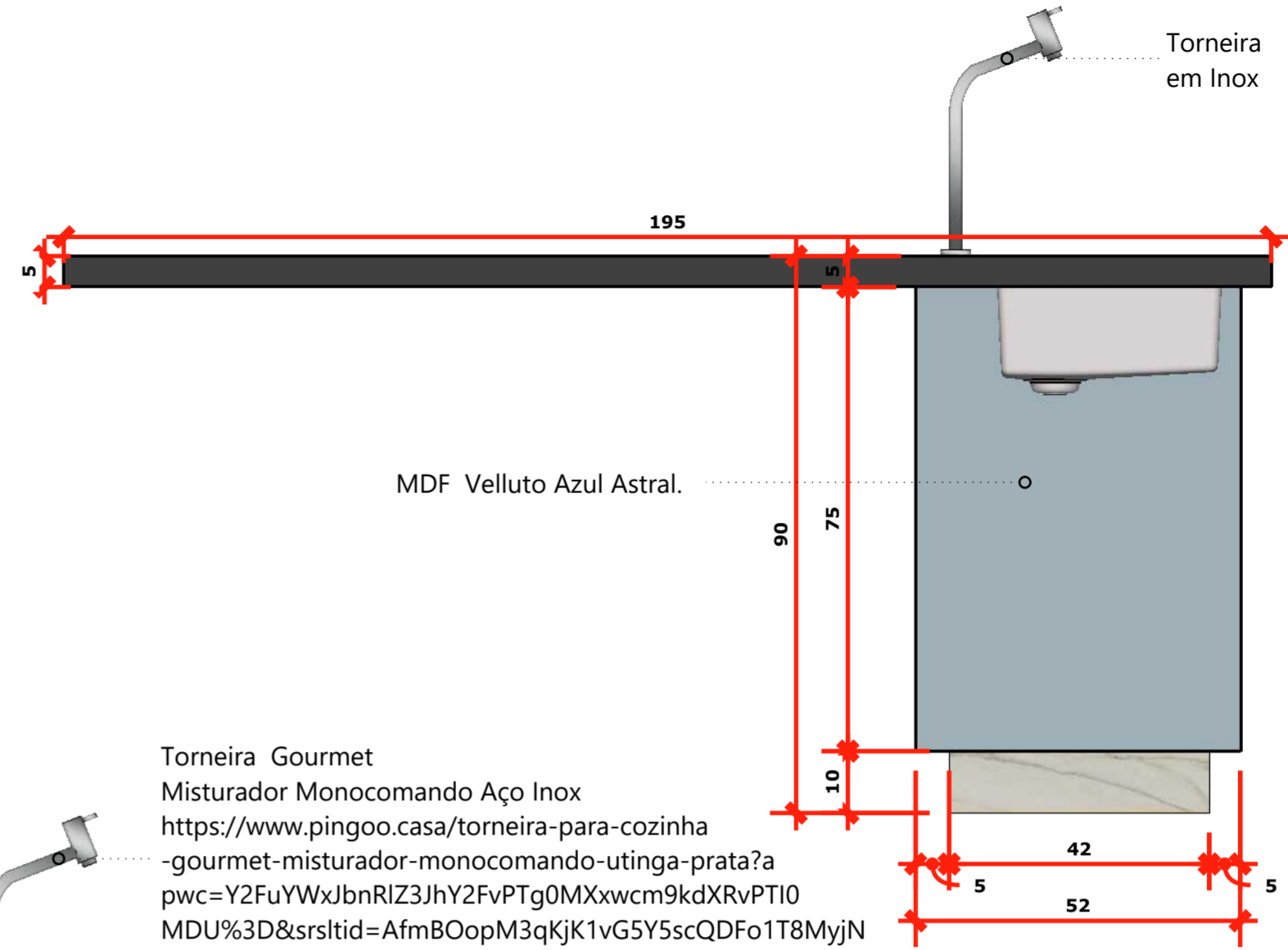
Vista Frontal ( corte ) - Bancada de experimentos
