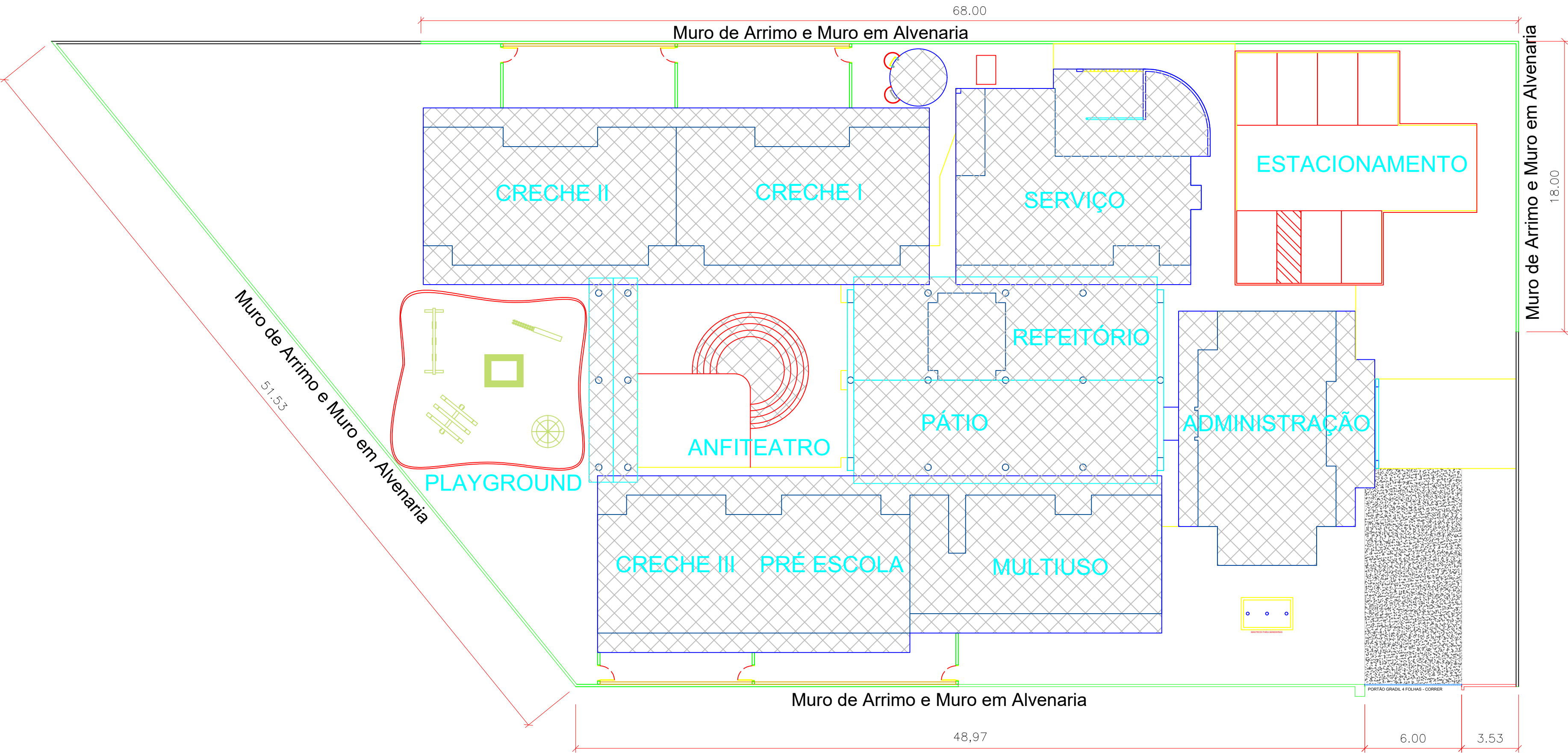
IMPLANTAÇÃO-MURO ESCALA:1/200
