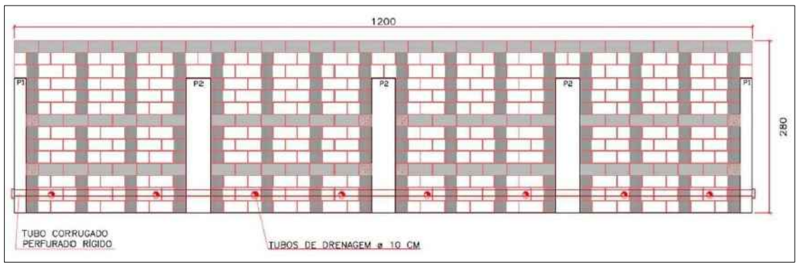
PROJETO TIPO - MURO DE ARRIMO (PADRÃO SINAPI) VISTA FRONTAL SEM ESCALA
