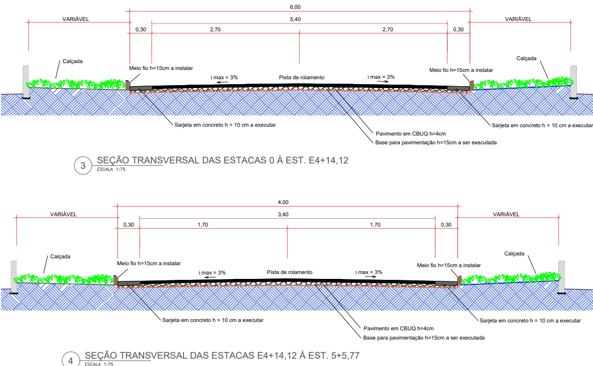
4 SEÇÃO TRANSVERSAL DAS ESTACAS E4+14,12 À EST. E5+5,77
