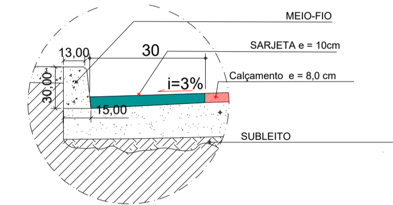
DETALHE B 1:75
