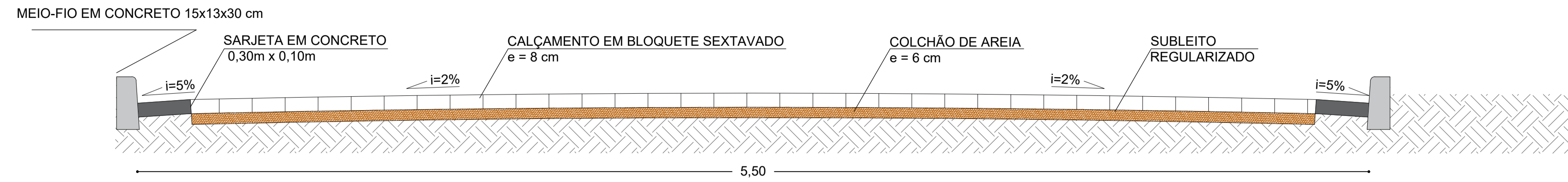
Corte Transversal 1:75
