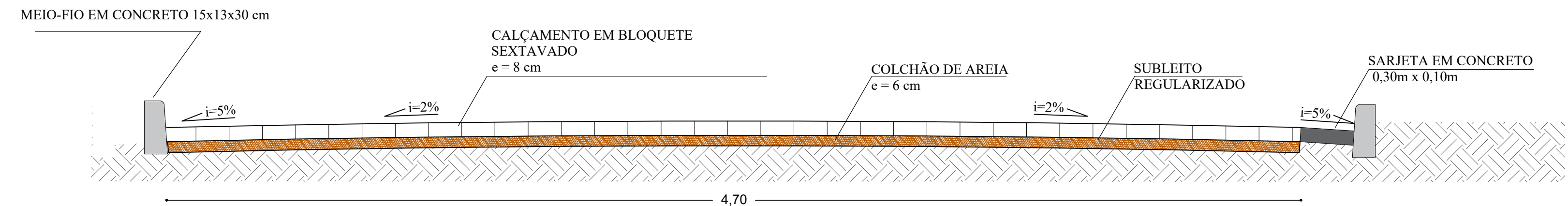
Corte Transversal 1:75
