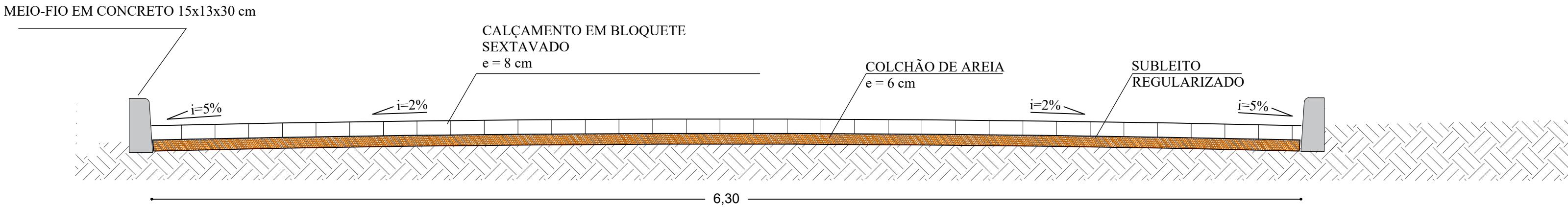
Corte Transversal 1:75
