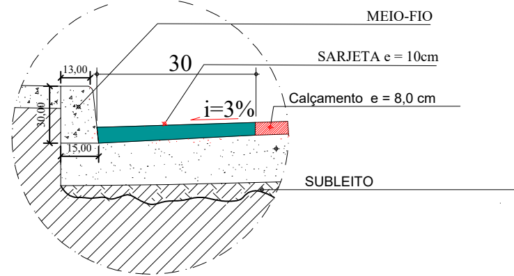
DETALHE B 1:75
