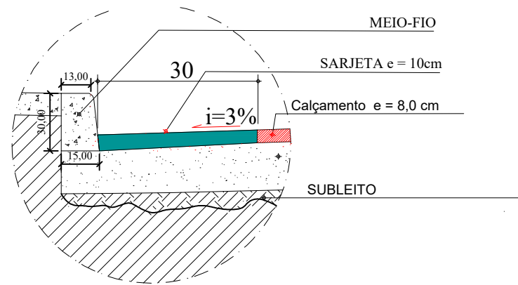
DETALHE B 1:75
