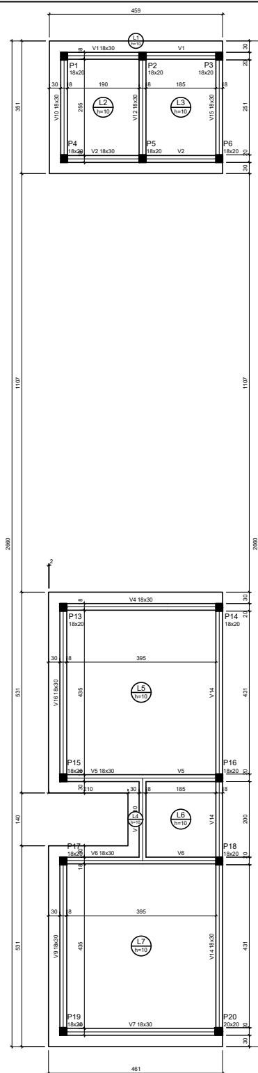
Forma Nível 300 escala 1:50
