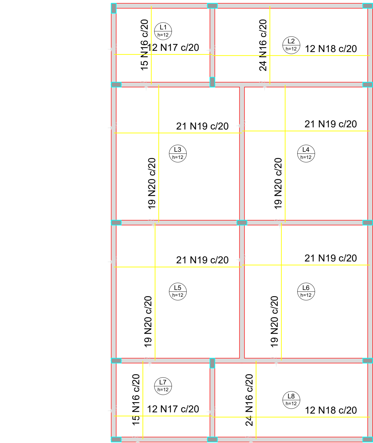
Armação positiva das lajes do pavimento TERREO escala 1:50
