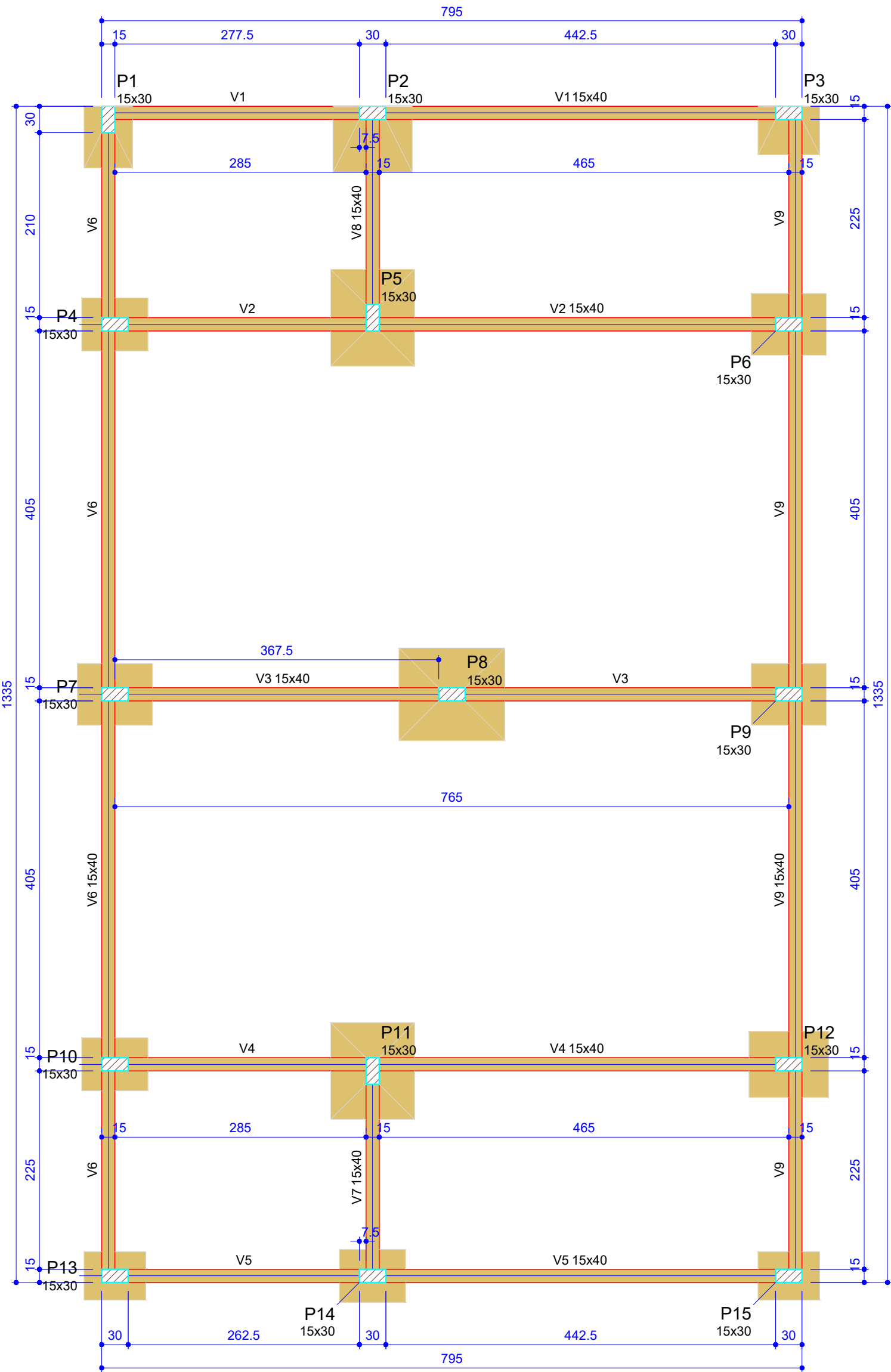
Forma do pavimento BALDRAME escala 1:50
