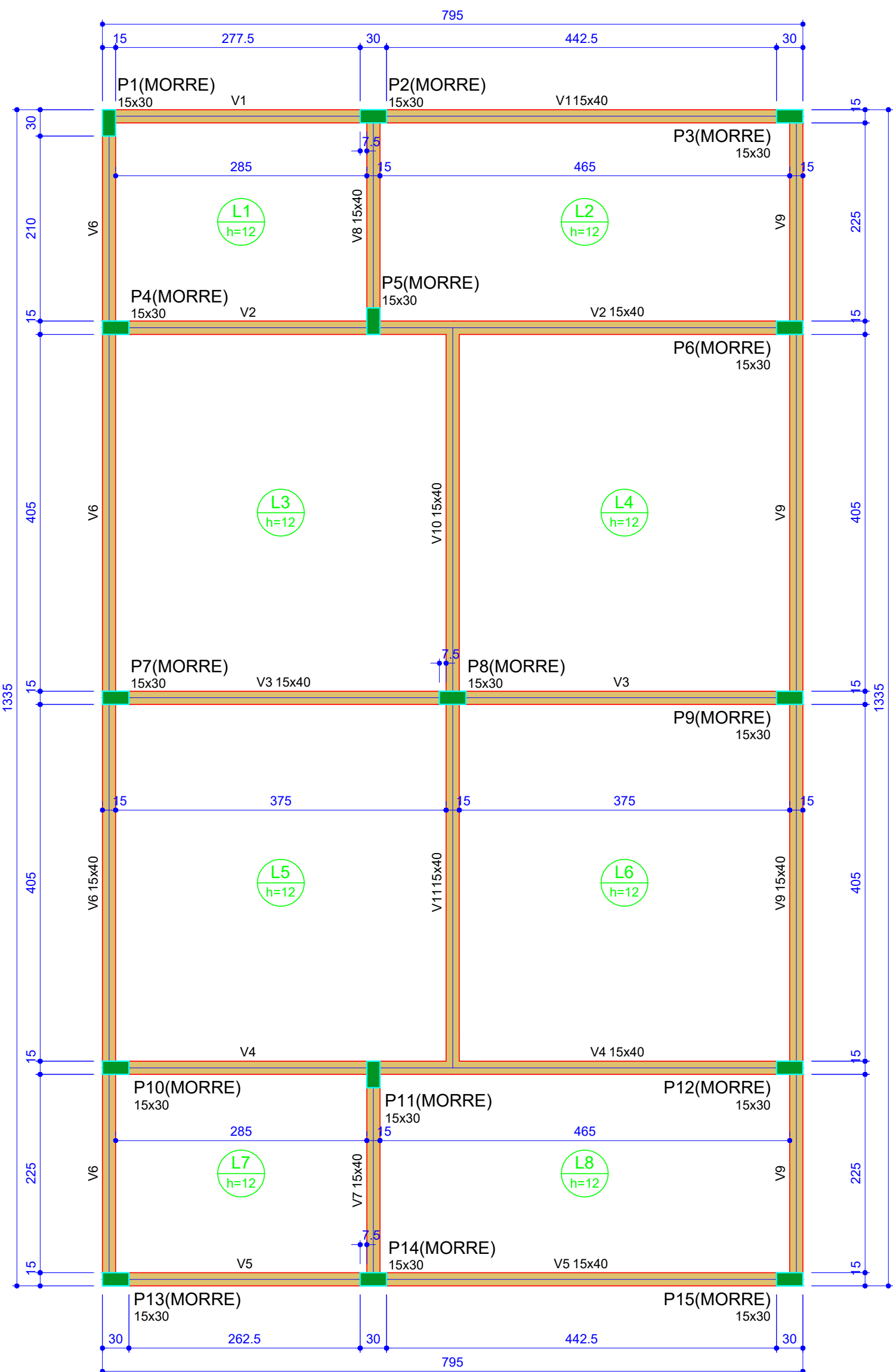
Forma do pavimento TERREO escala 1:50
