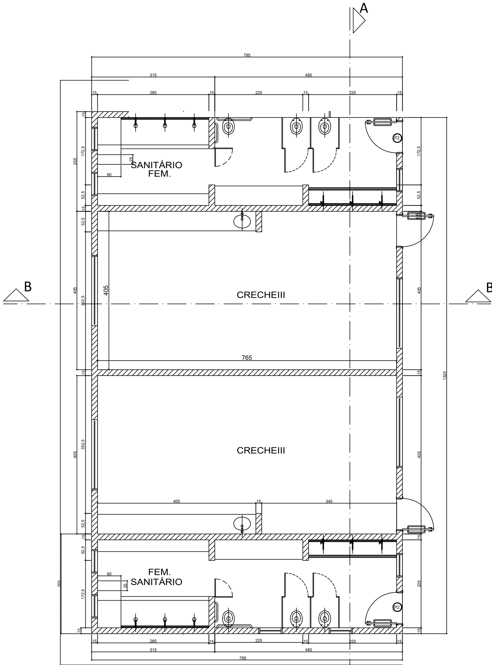
PLANTA BAIXA esc 1:100
