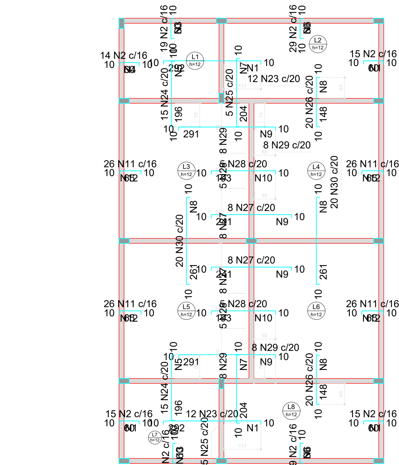
Armação negativa das lajes do pavimento TERREO escala 1:50
