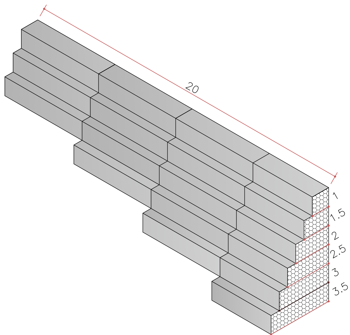
PERSPECTIVA ISOMÉTRICA DO GABIÃO Sem escala
