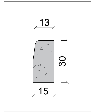
DETALHE - MEIO-FIO Sem escala
