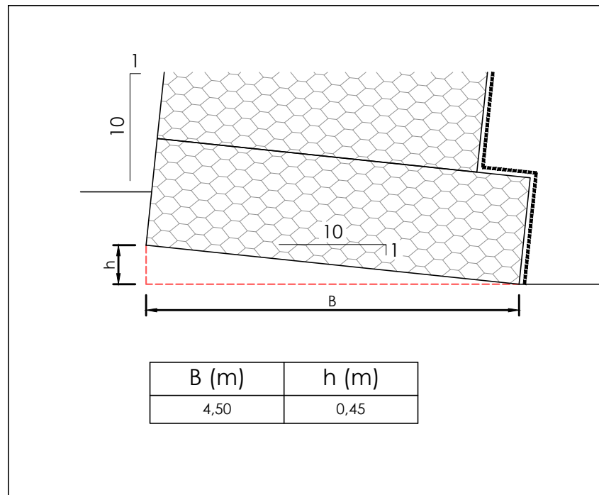
DETALHE PREPARAÇÃO DA BASE Sem escala
