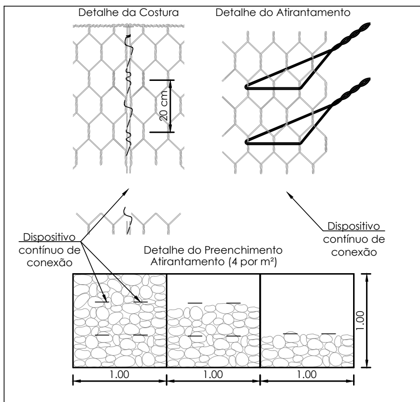
DETALHE AMARRAÇÃO DA MALHA Sem escala
