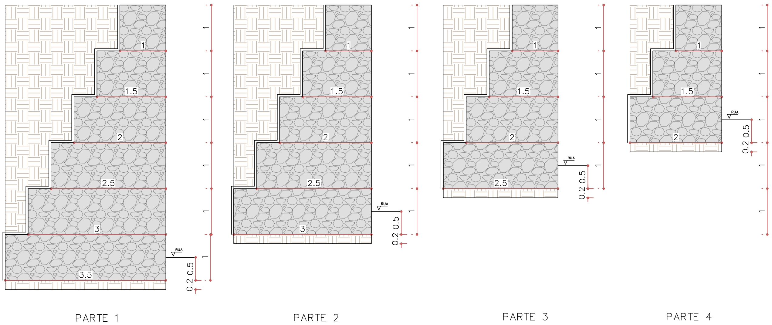
COMPOSIÇÃO GABIÃO Escala 1:50
