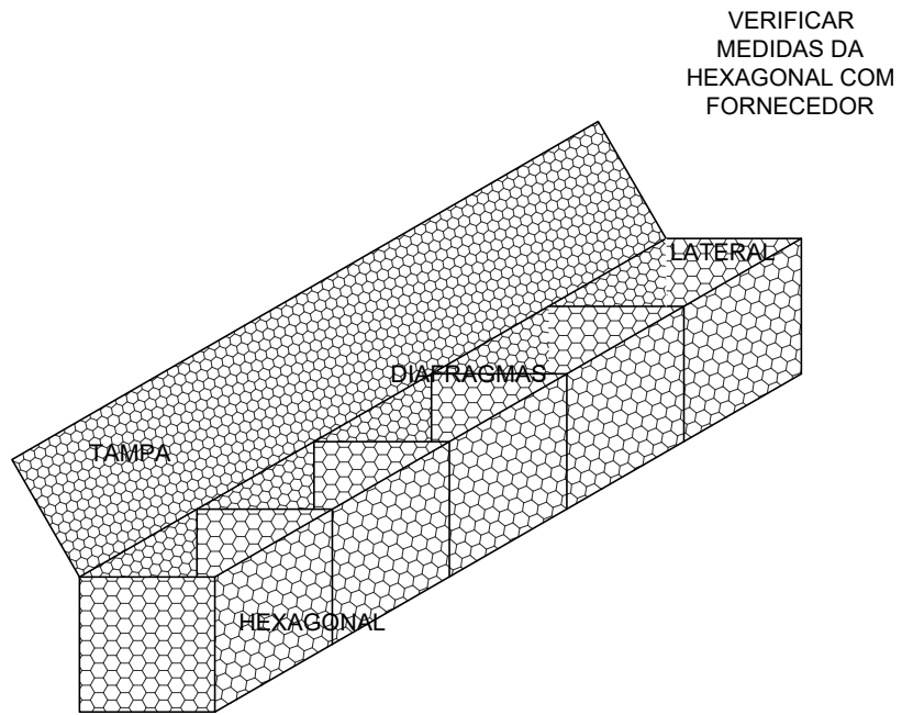
PERSPECTIVA ISOMÉTRICA CAIXA DE GABIÃO Sem escala
