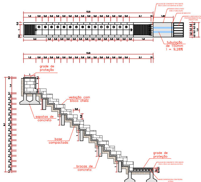
DETALHE - ESCADA HIDRAULICA Sem escala
