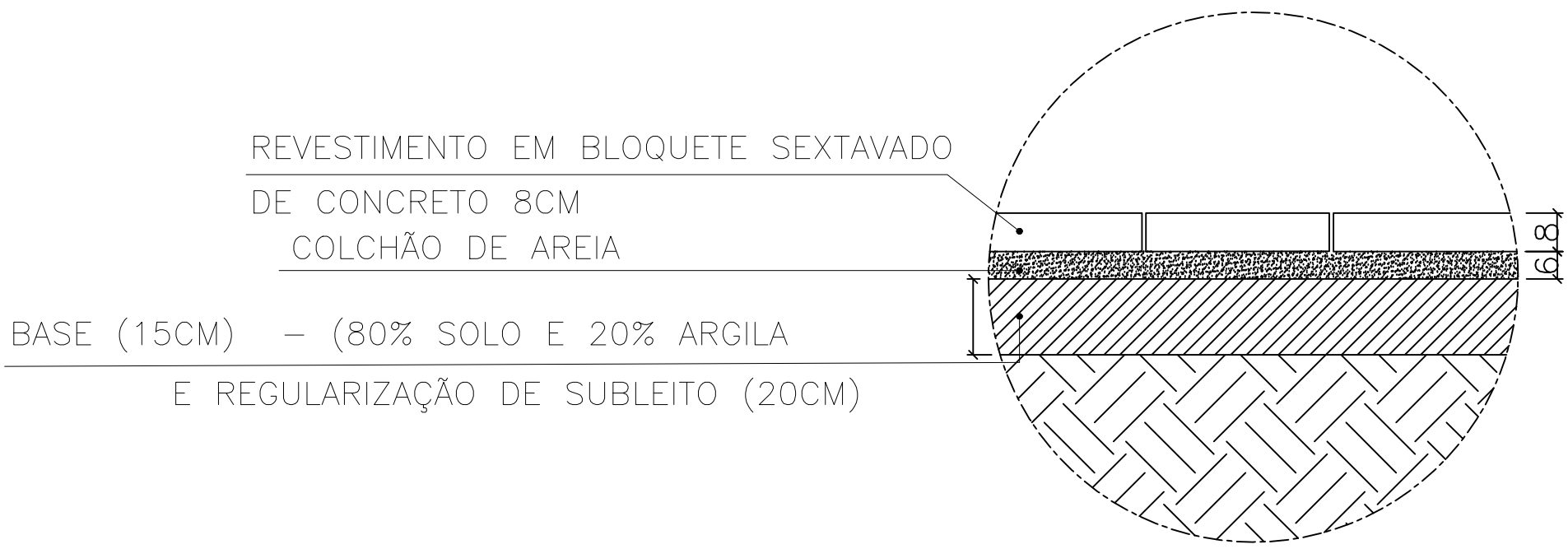
DET. 02 SEM ESCALA CAMADAS DO CALÇAMENTO
