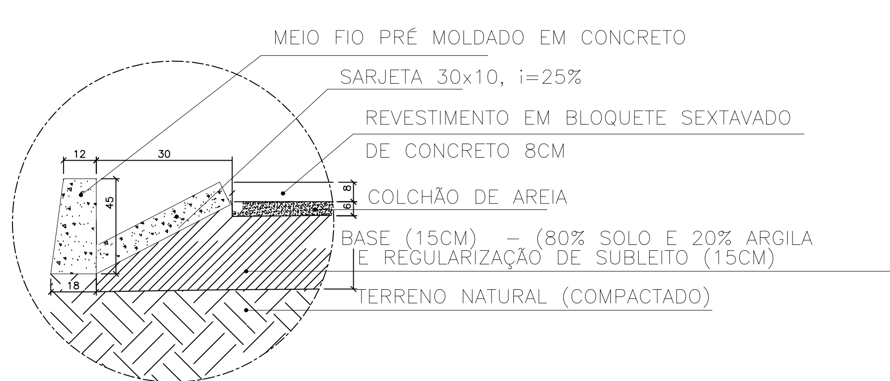
DET. 01 SEM ESCALA DETALHES DO CALÇAMENTO
