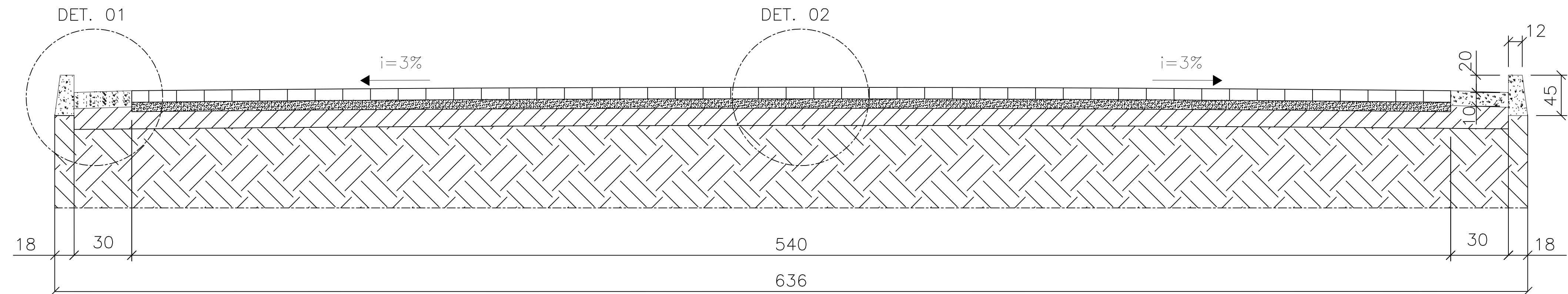
SEÇÃO TRANSVERSAL BÁSICA DAS VIAS SEM ESCALA
