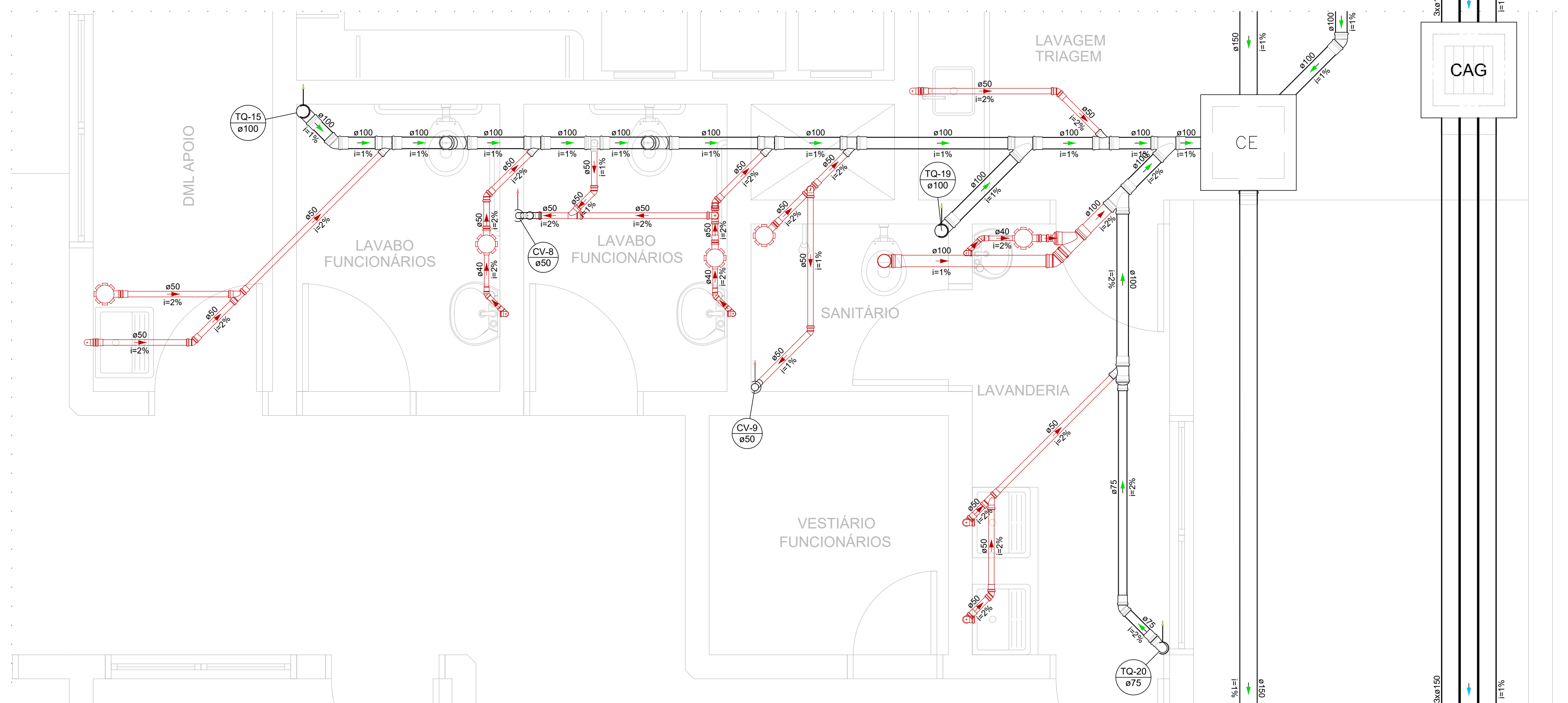
Detalhe S9 Escala 1:25
