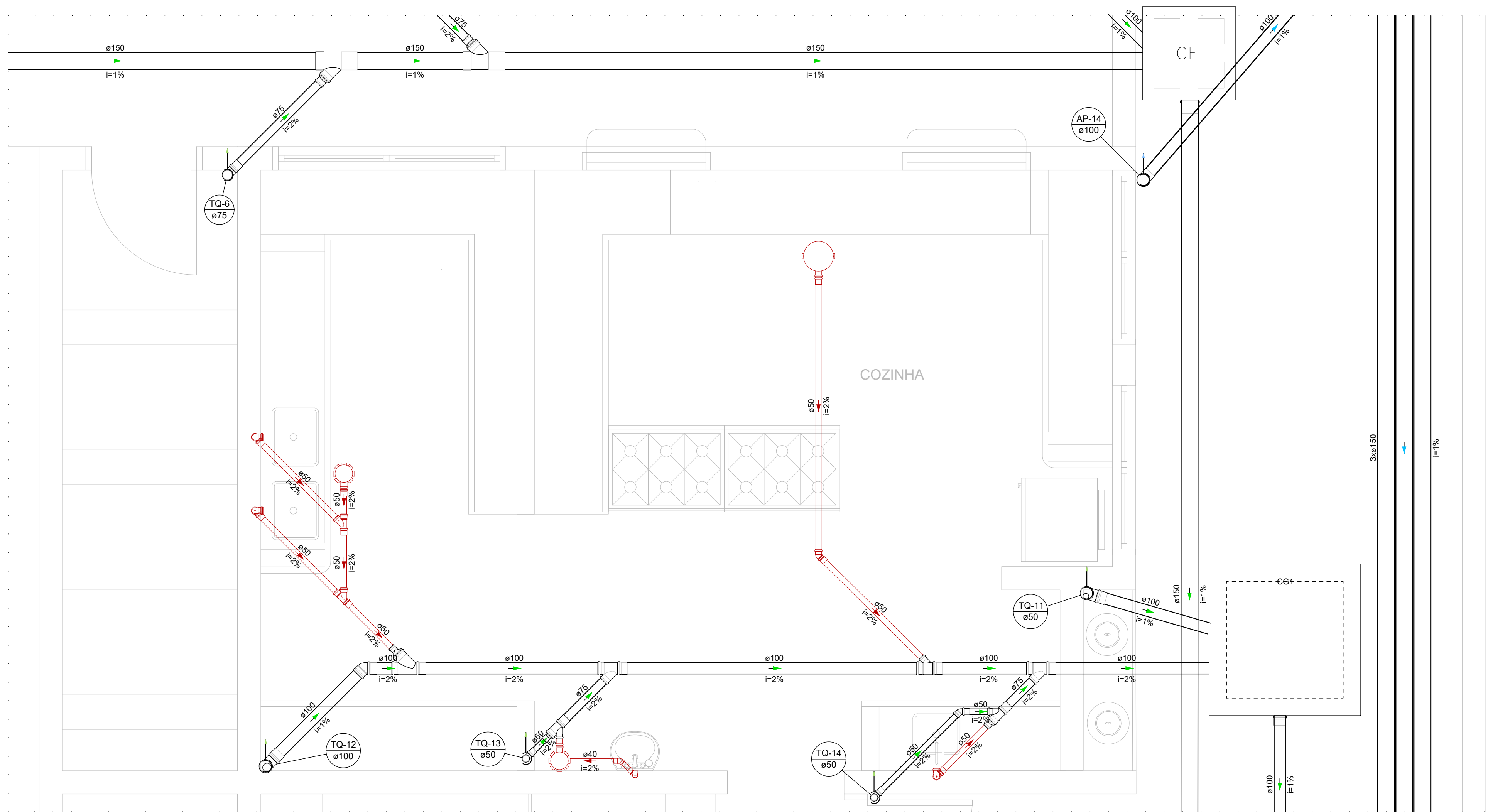
Detalhe S3 Escala 1:25
