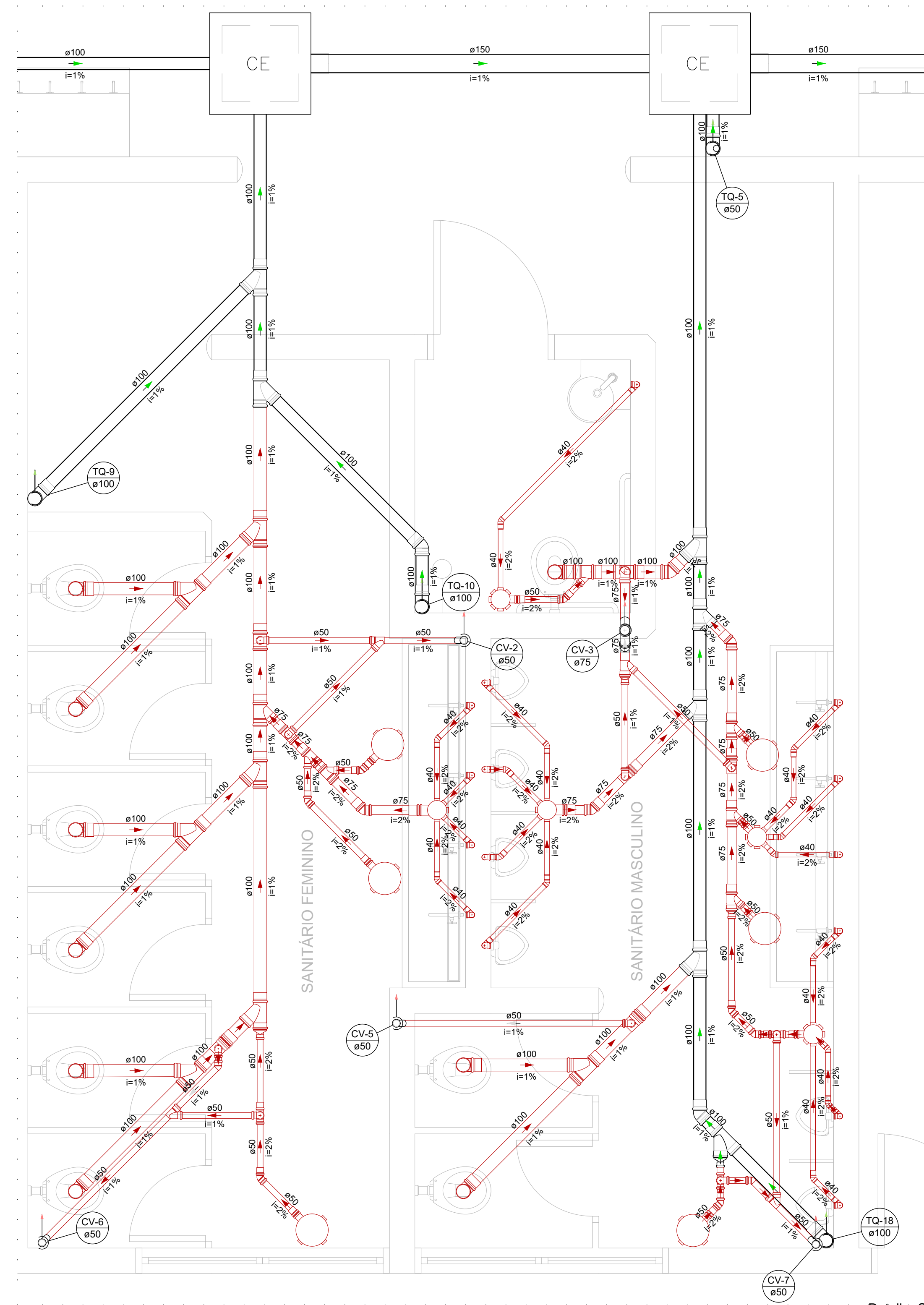
Detalhe S5 Escala 1:25
