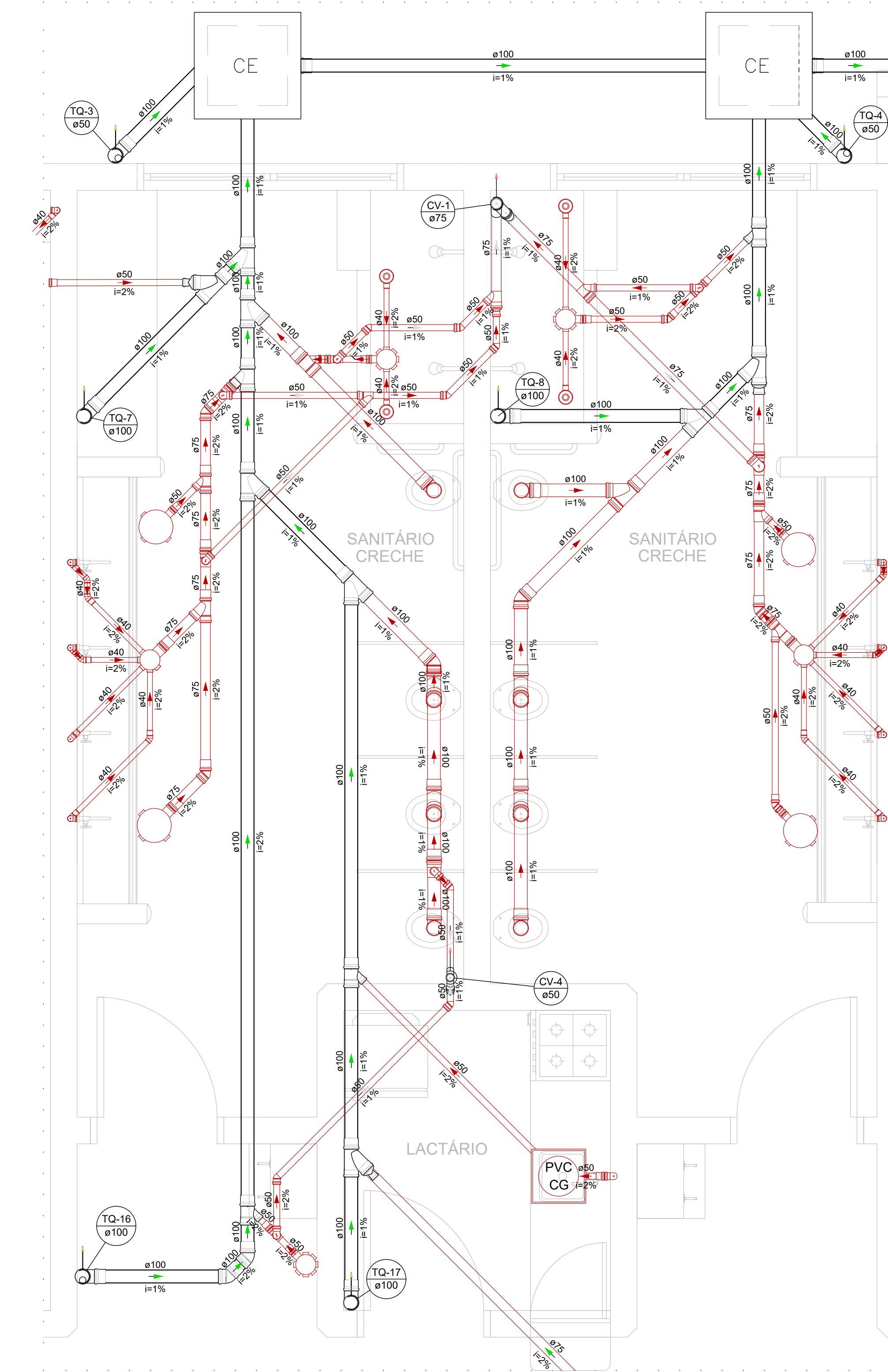
Detalhe S4 Escala 1:25
