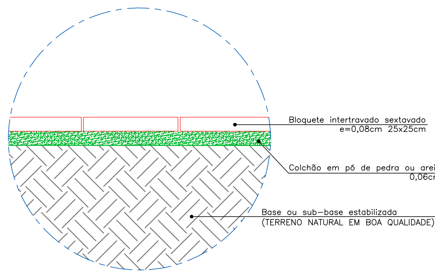
Det. 02 - Calçamento Sem escala
