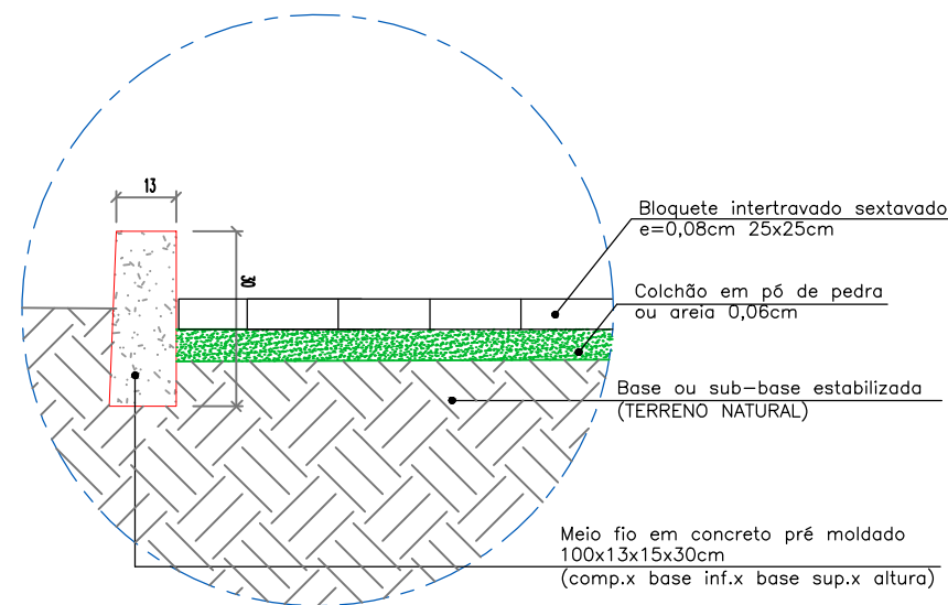
Det. 01 - Meio fio Sem escala
