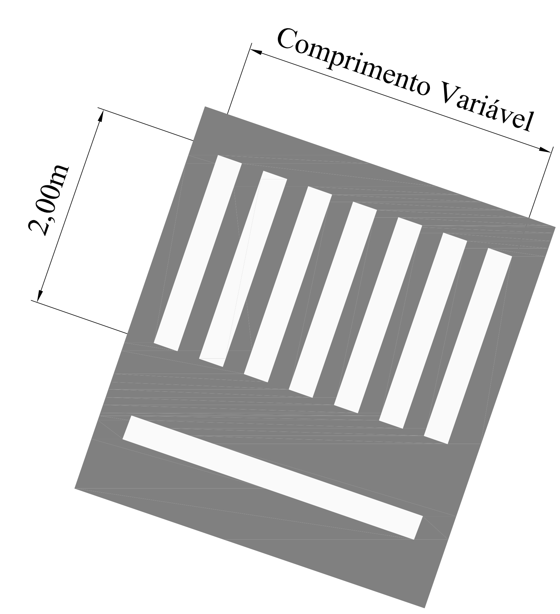
DIMENSIONAMENTO DA FAIXA DE PEDRESTE
