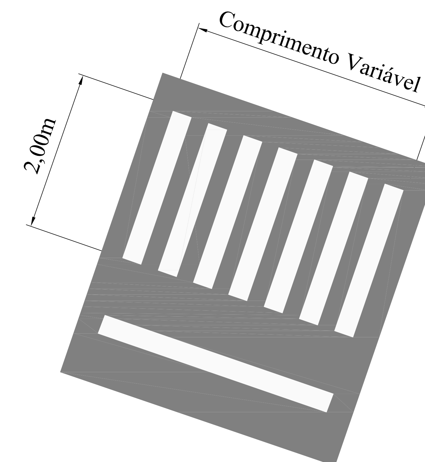
DIMENSIONAMENTO DA FAIXA DE PEDRESTE
