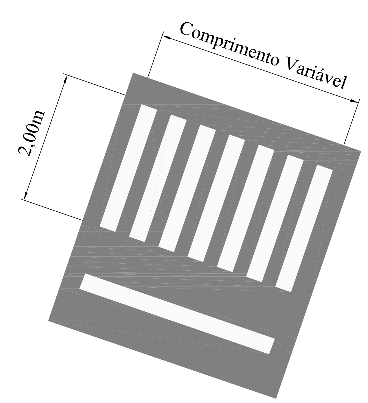
DIMENSIONAMENTO DA FAIXA DE PEDRESTE
