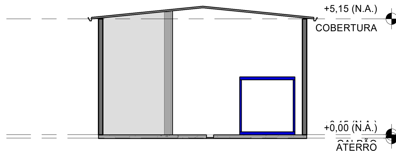
4 CORTE AA 1 : 100
