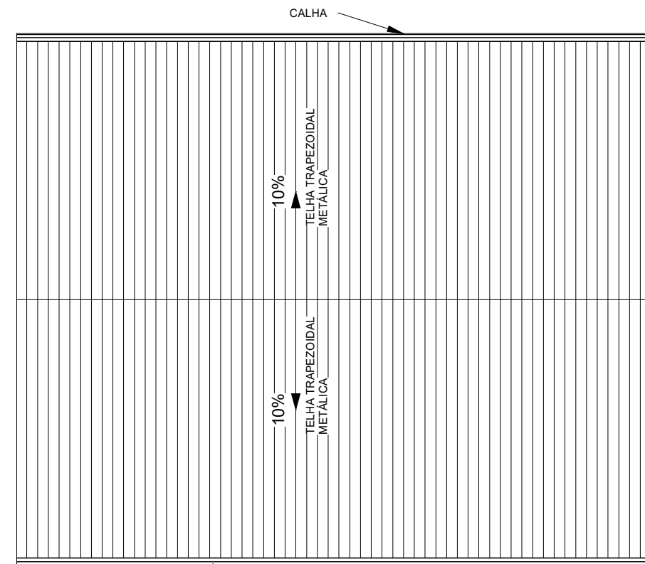
2 COBERTURA 1 : 100
