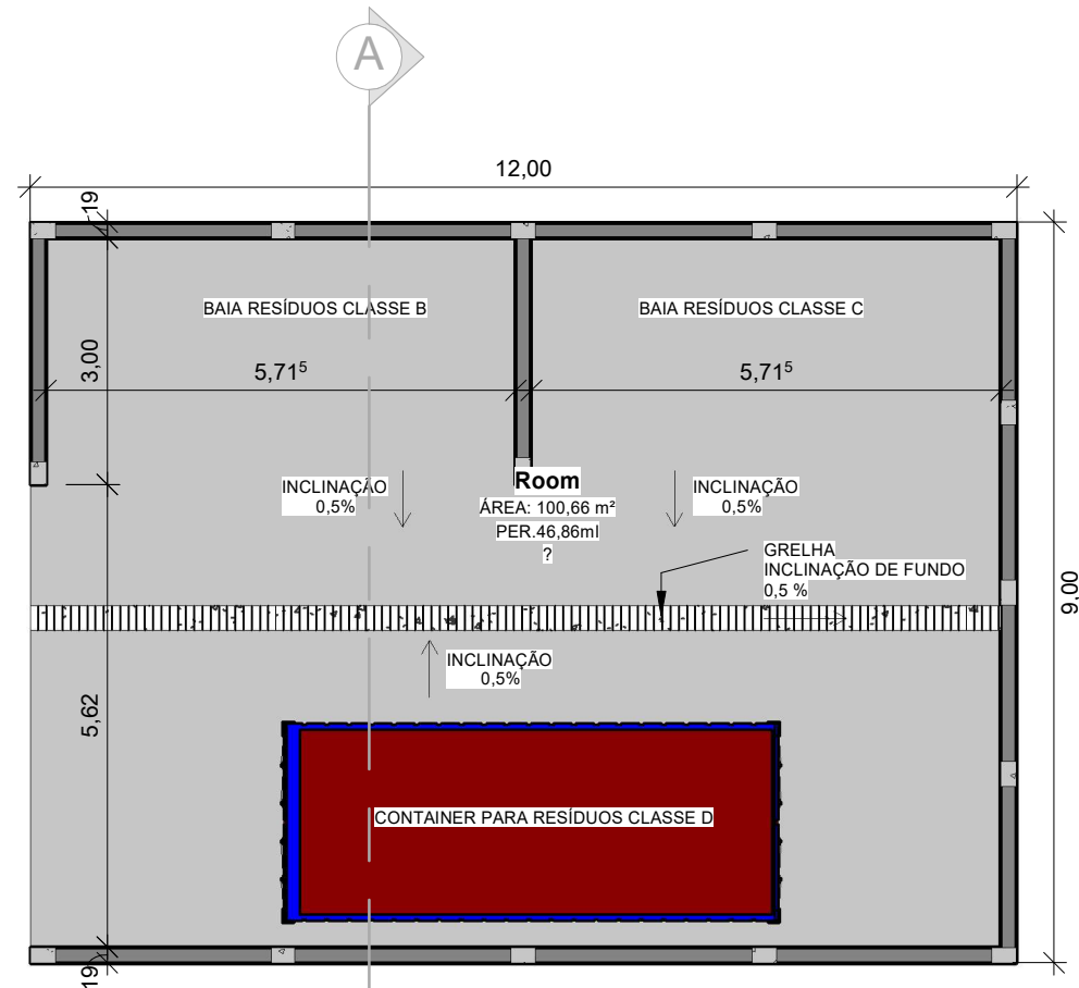
1 PLANTA BAIXA 1 : 100
