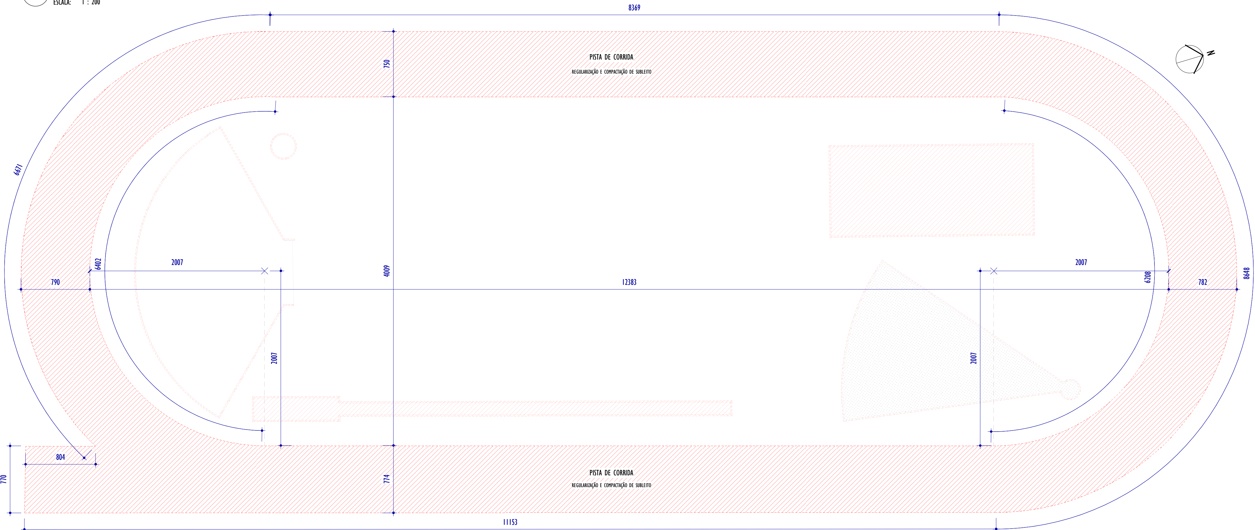
2 PISTA DE ATLETISMO - PLANTA DE DEMOLIÇÃO
