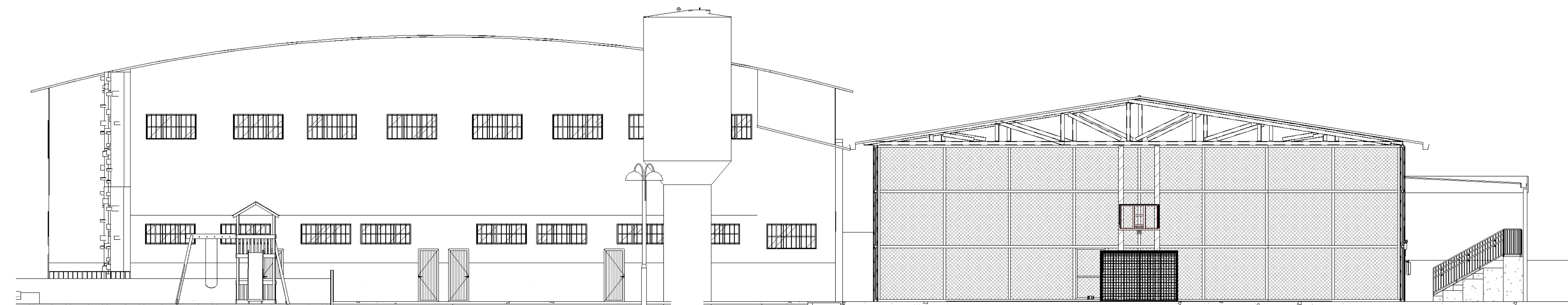
2 FACHADA POSTERIOR 1 : 100
