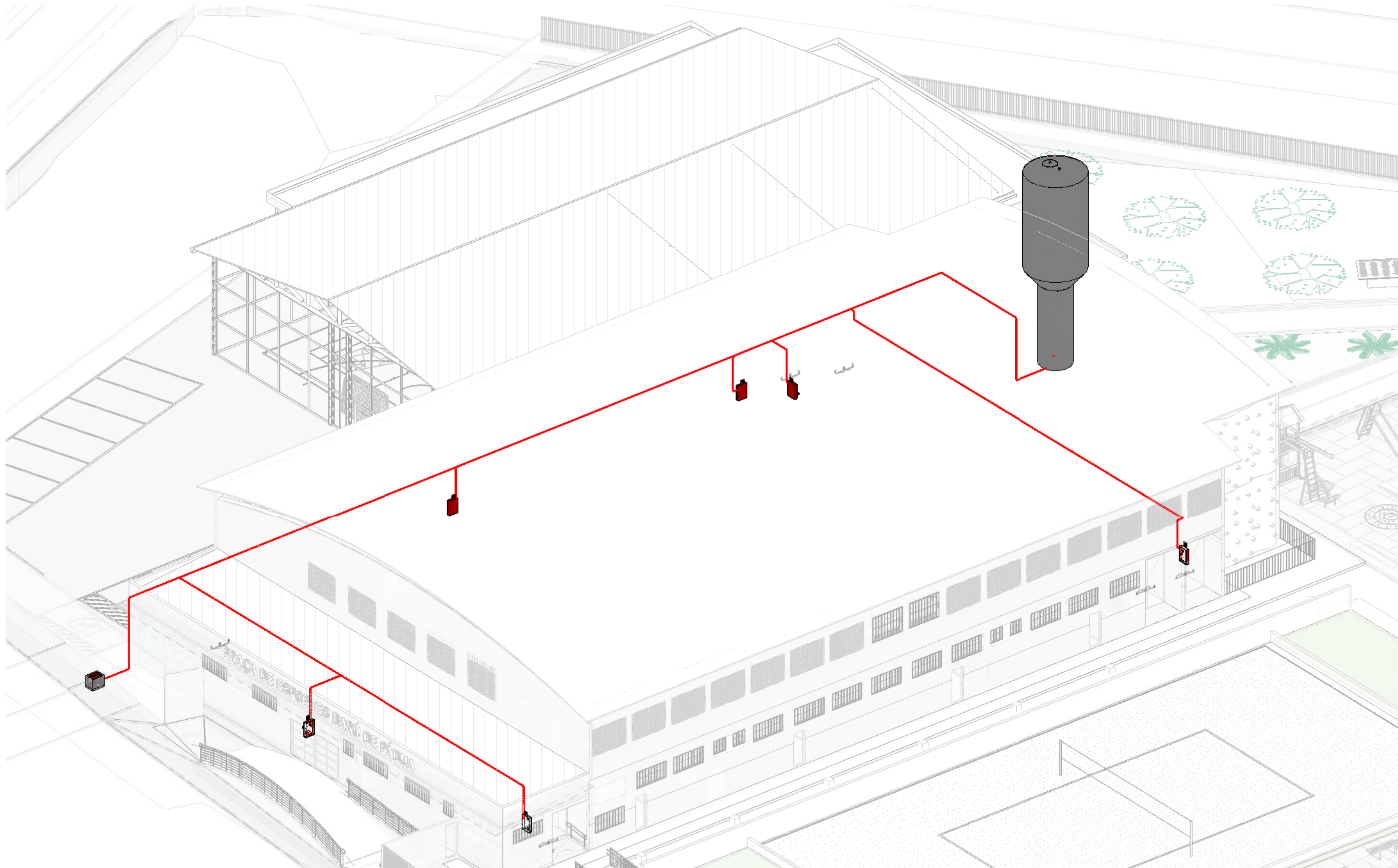
2 ISOMÉTRICO HIDRANTE
