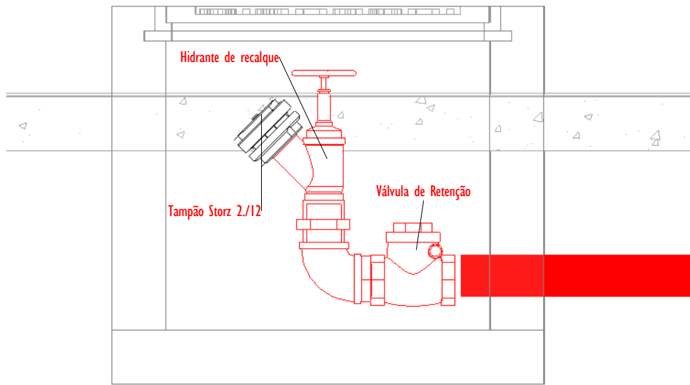
2 DETALHE RECALQUE ESCALA: 1 : 10
