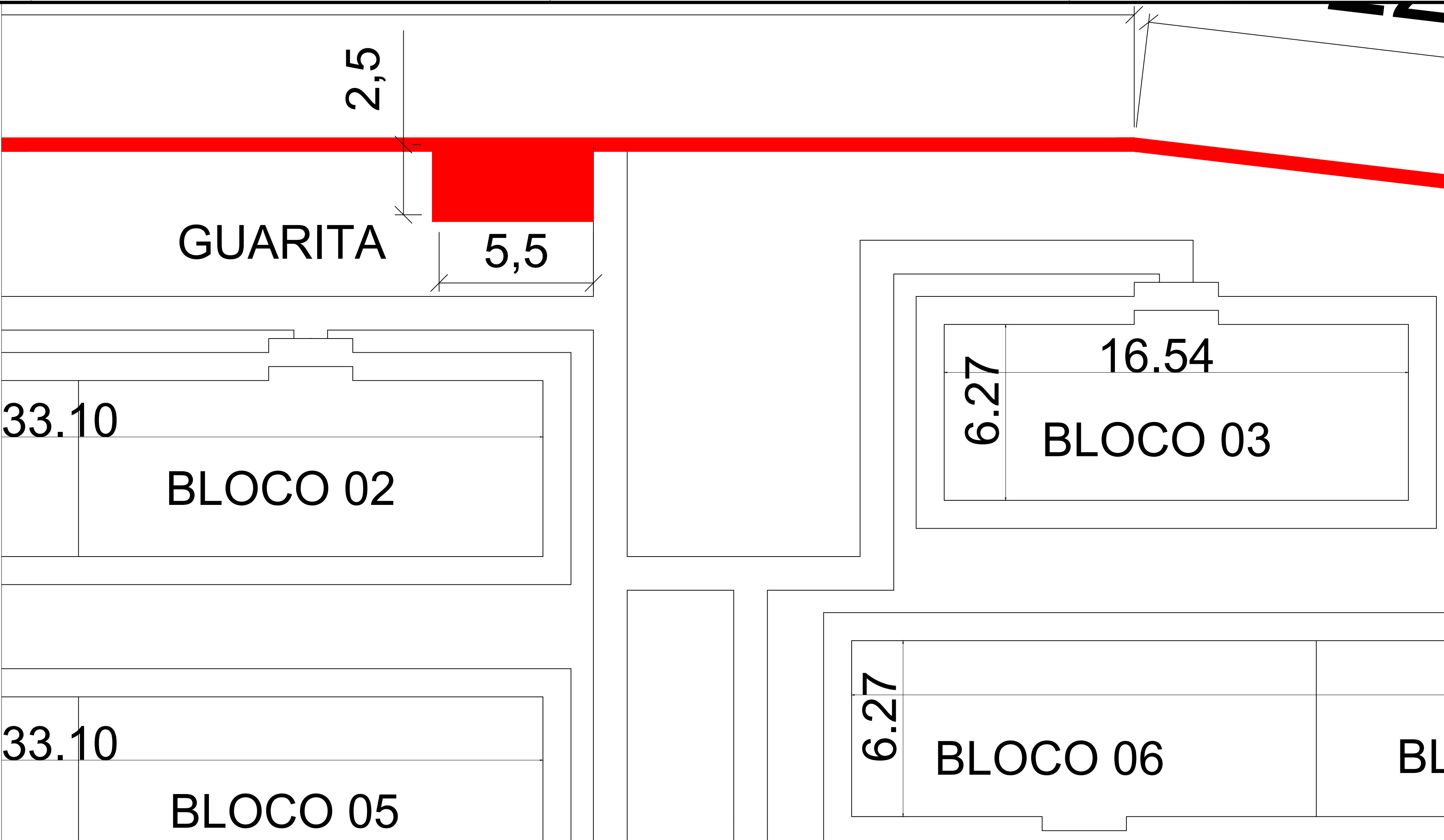
DETALHE: GUARITA A SER DEMOLIDA ESC 1/100
