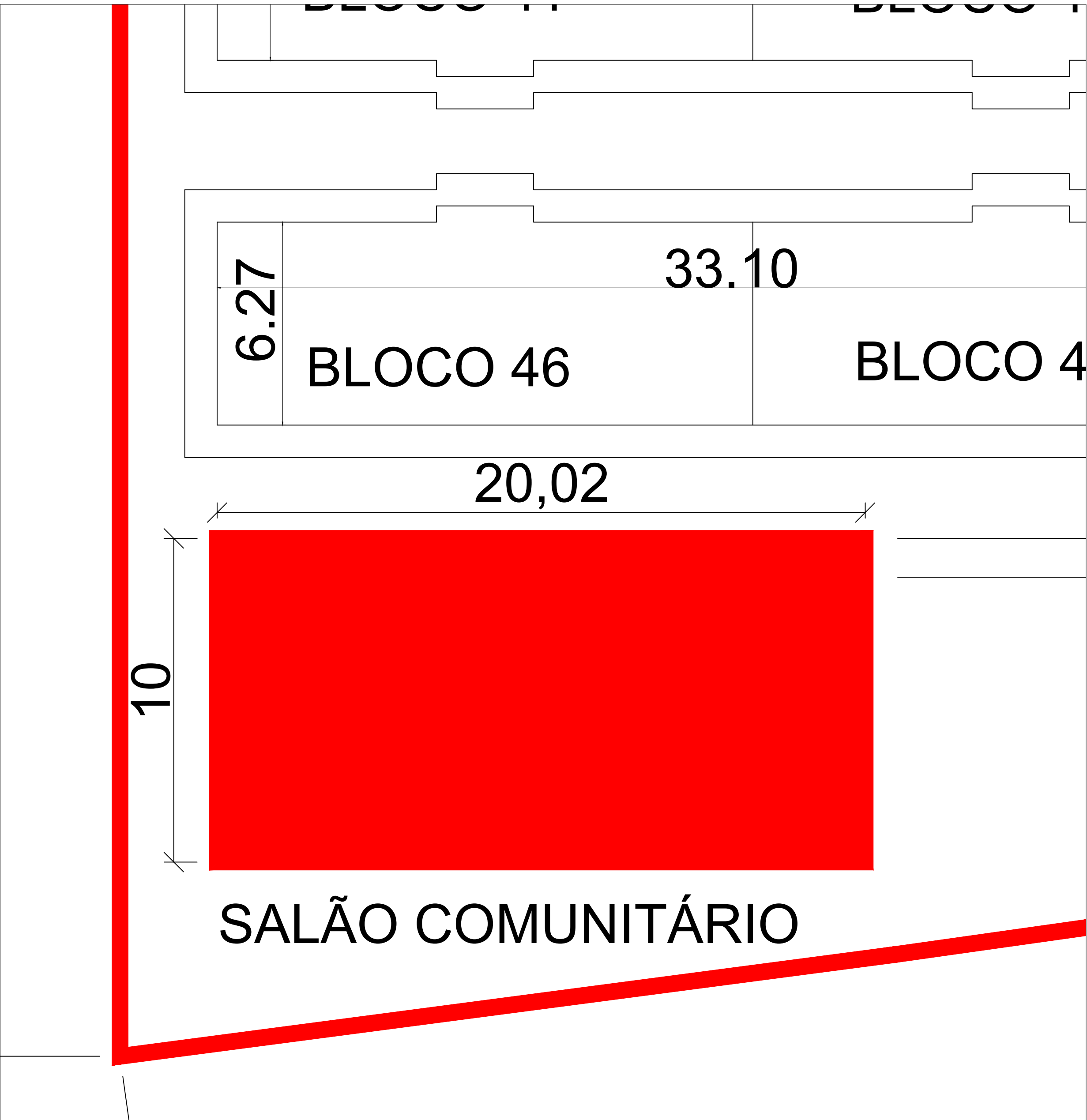
DETALHE: BARRACÃO A SER DEMOLIDO ESC 1/100
