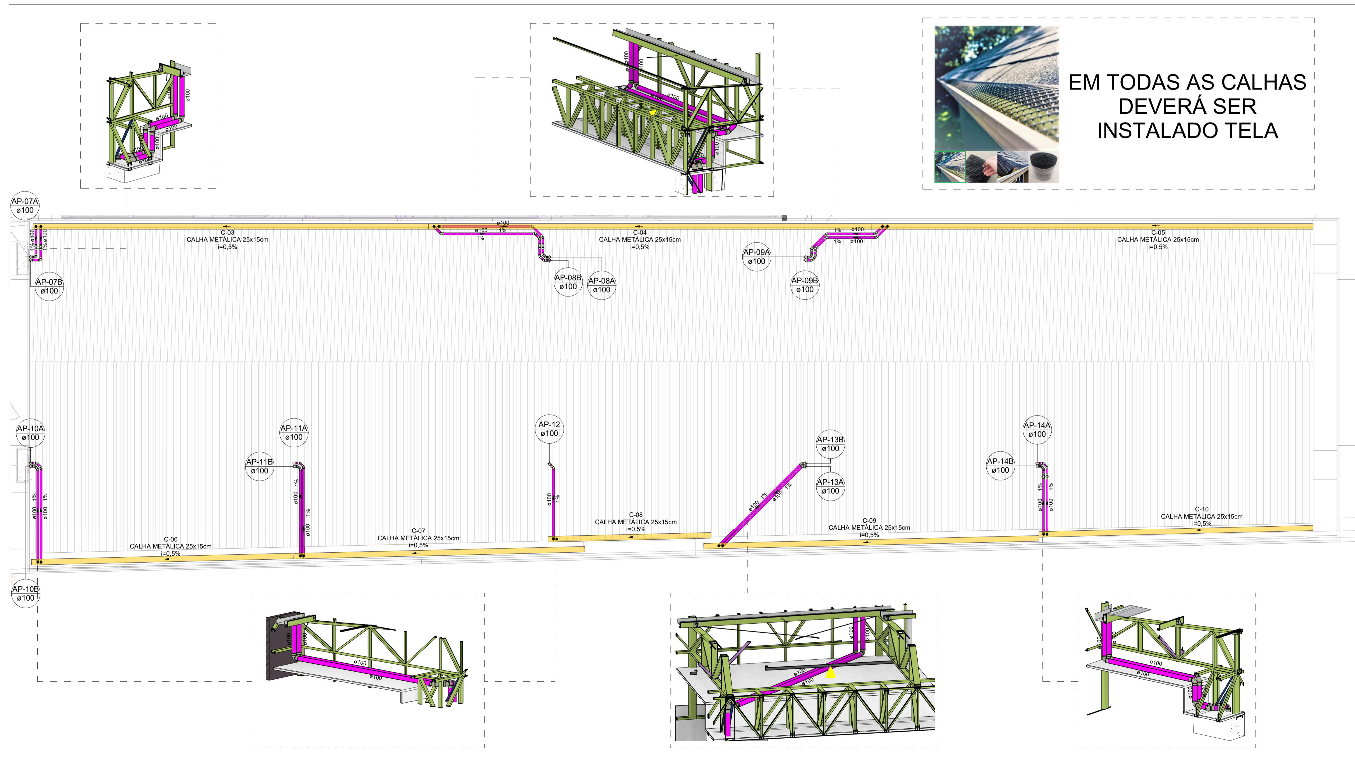
PLANTA BAIXA REDE DE DRENAGEM PLUVIAL - COBERTURA METÁLICA
