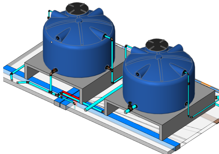
Tanque polietileno 3d - 3.000 litros
