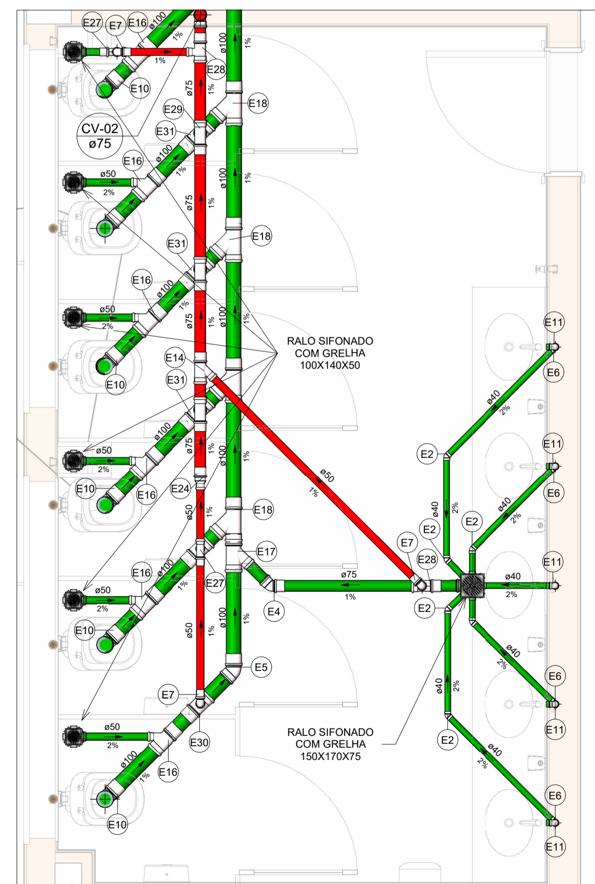
SAN-04 Escala 1 : 25
