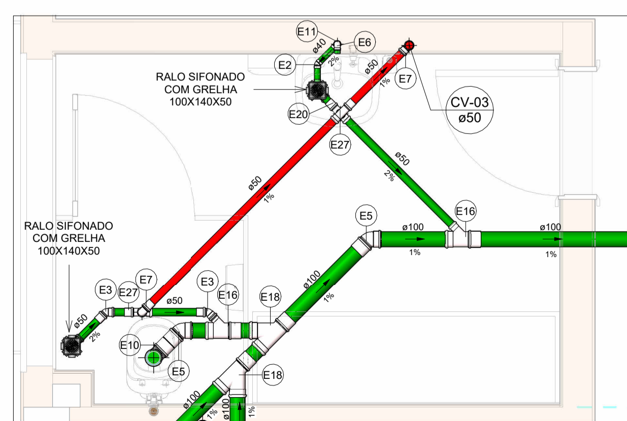
SAN-05 Escala 1 : 25
