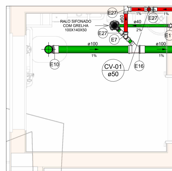
SAN-01 Escala 1 : 25
