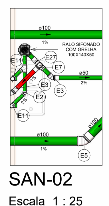
SAN-02 Escala 1 : 25
