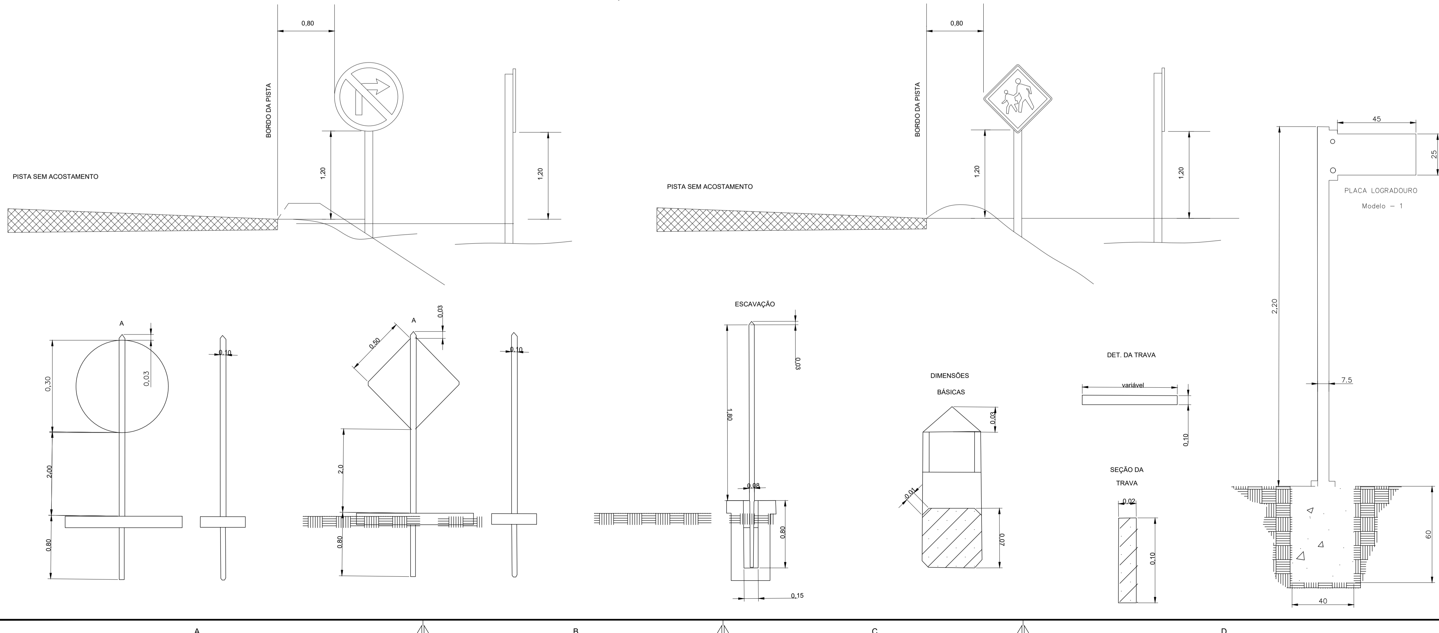
ESQUEMA DE INSTALAÇÃO DE PLACAS
