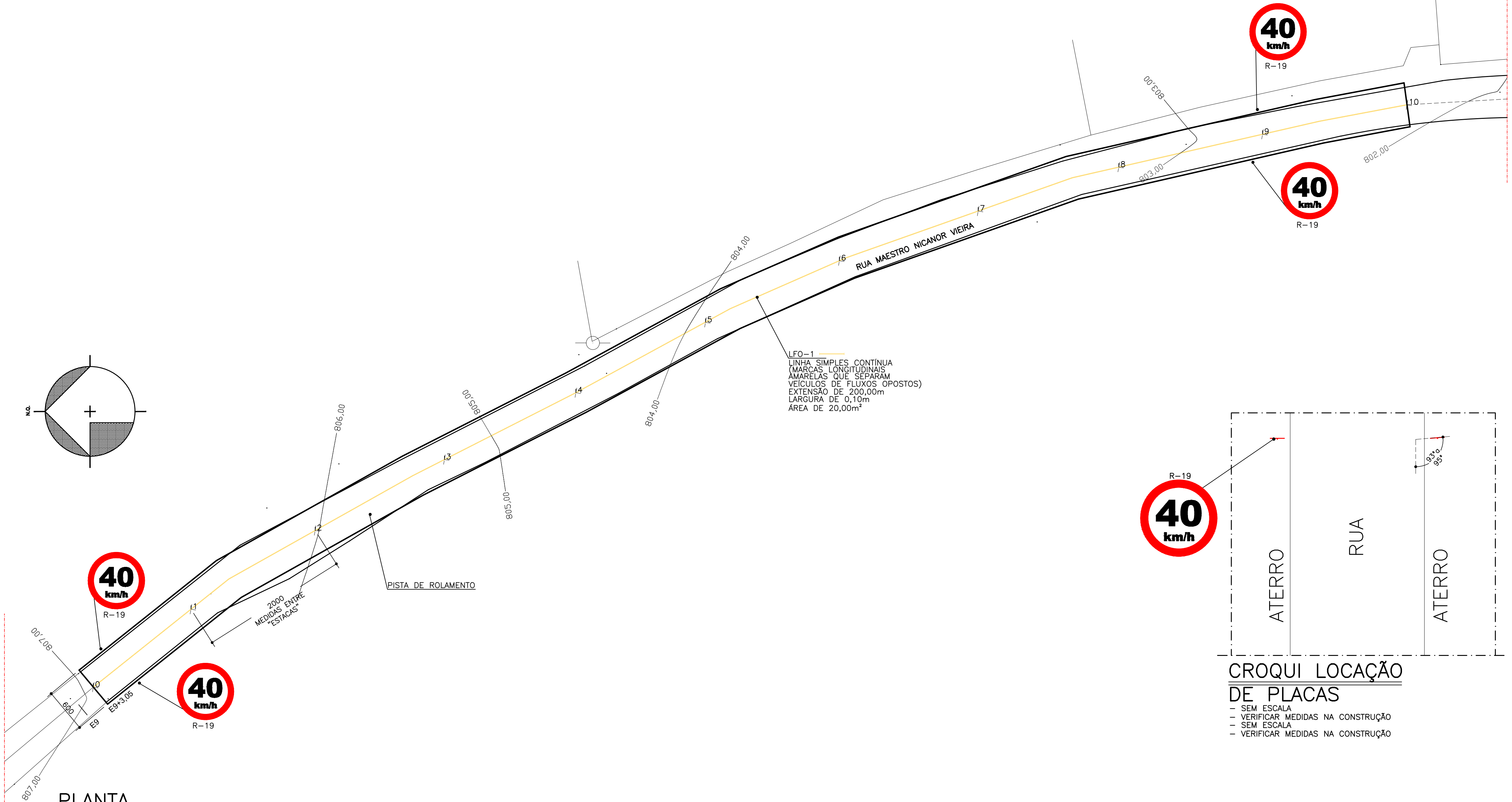
PLANTA SINALIZAÇÃO - ESC.: 1/325 - LINHAS DE COTA EM CENTÍMETROS - VERIFICAR MEDIDAS NA CONSTRUÇÃO
