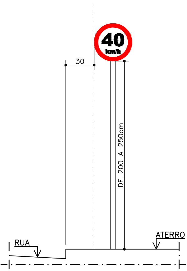
ELEVÇÃO R-19 - SEM ESCALA - DIÂMETRO DA PLACA = 0,40m - VERIFICAR MEDIDAS NA CONSTRUÇÃO
