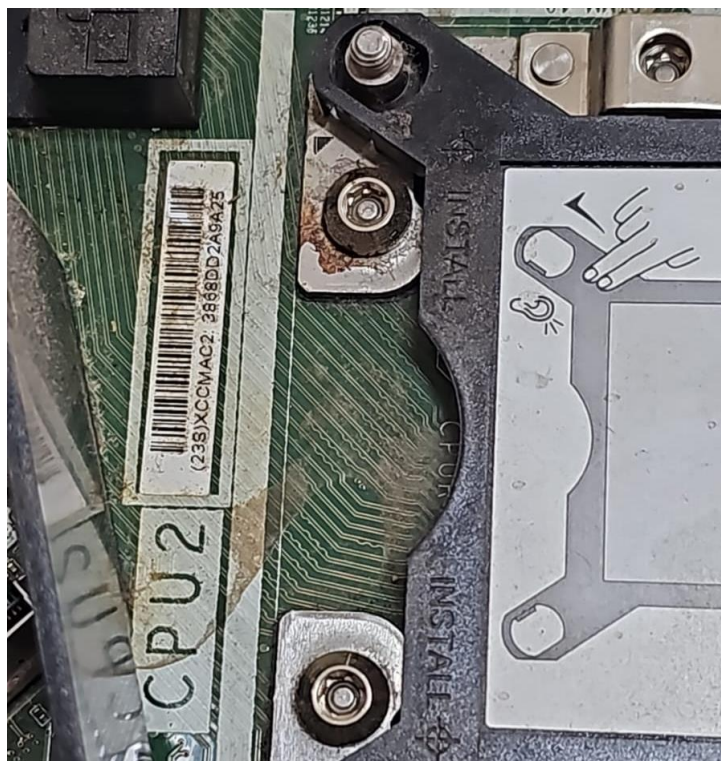
Figura 14: imagem das marcas de água na placa de circuito do servidor
