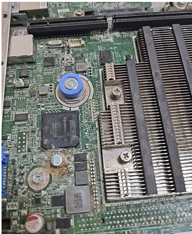
Figura 13: imagem das marcas de água na placa de circuito do servidor
