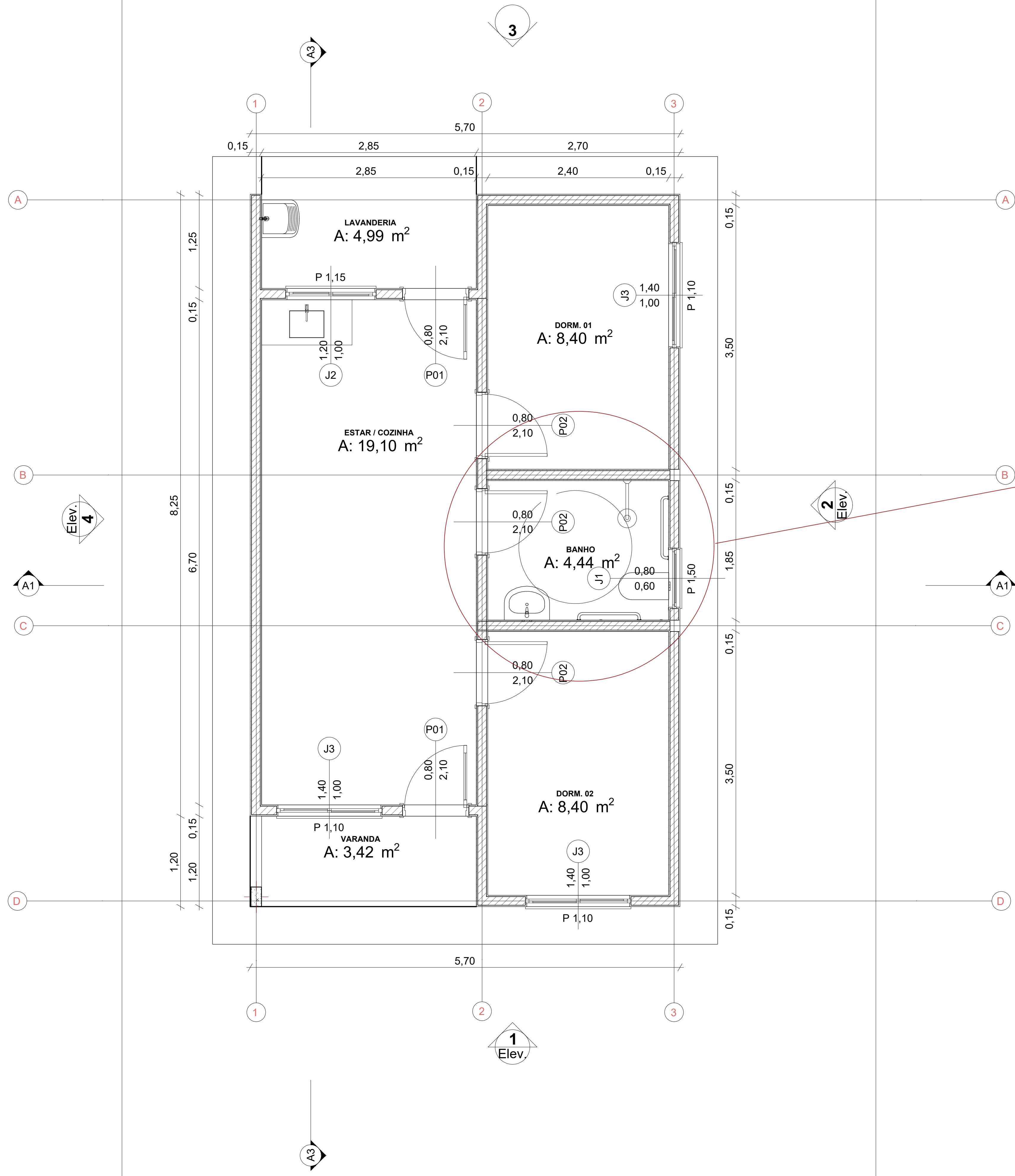
Planta Térreo 1:50
