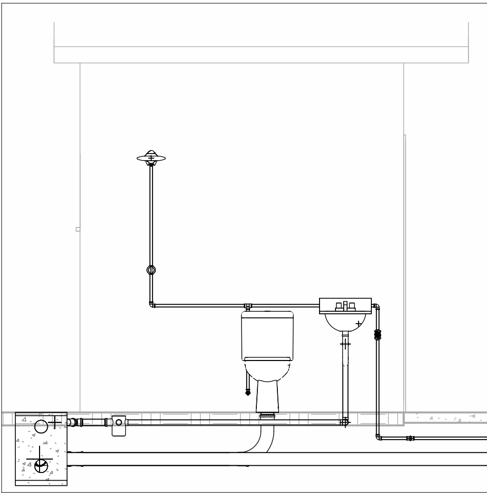
3 Corte B 1 : 30
