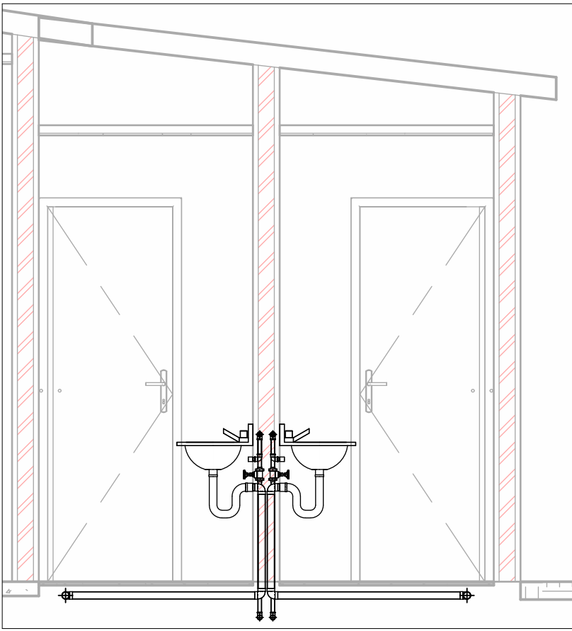
2 Corte A 1 : 30
