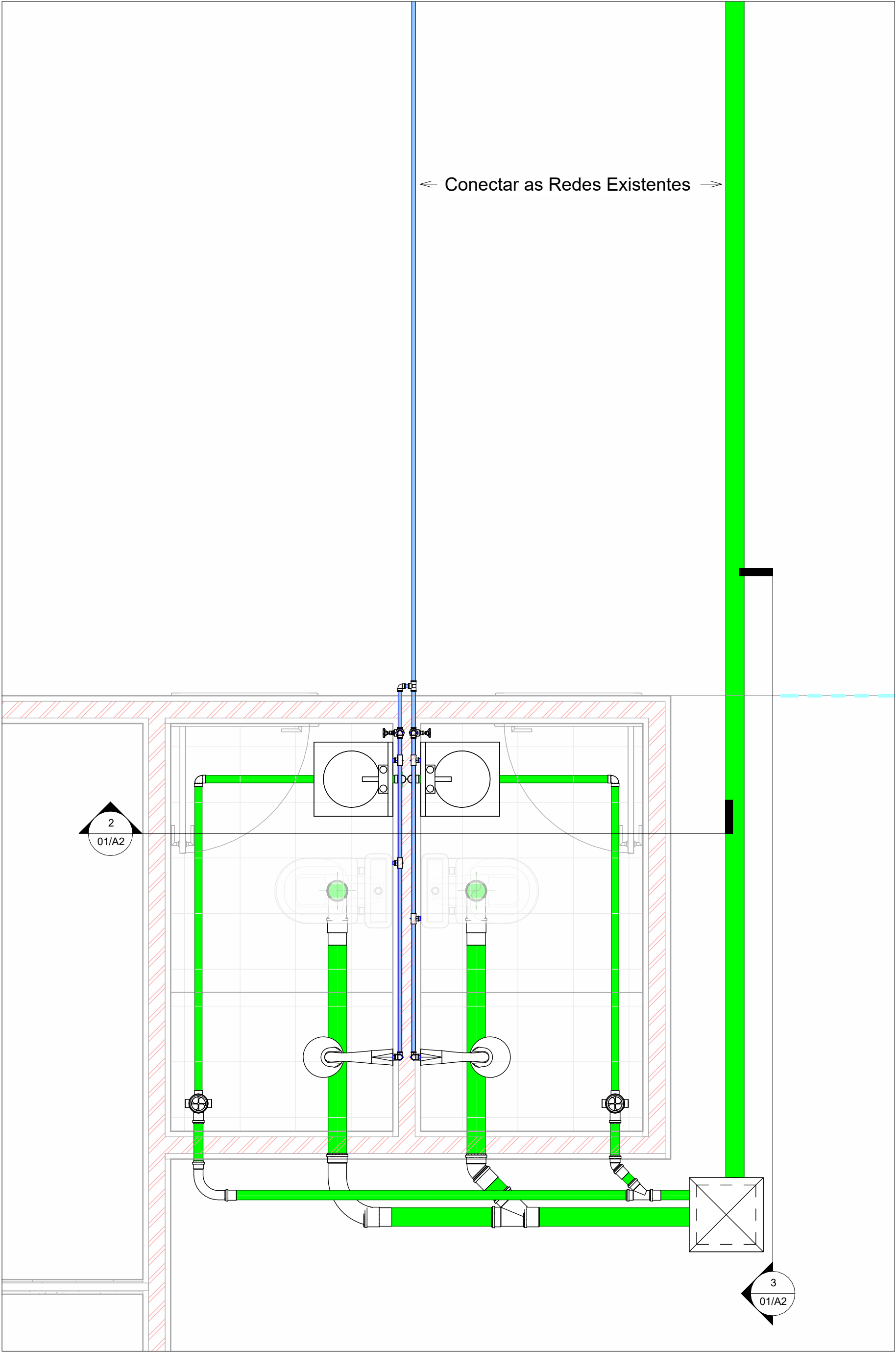
1 Planta Baixa 1 : 20
