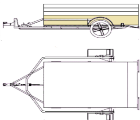
Figura 3 - carretinha basculante vedada.
