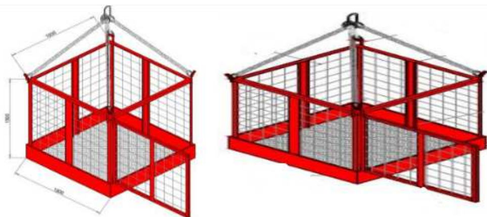
Figura 2. Modelo gaiola para transporte de materiais recicláveis.
