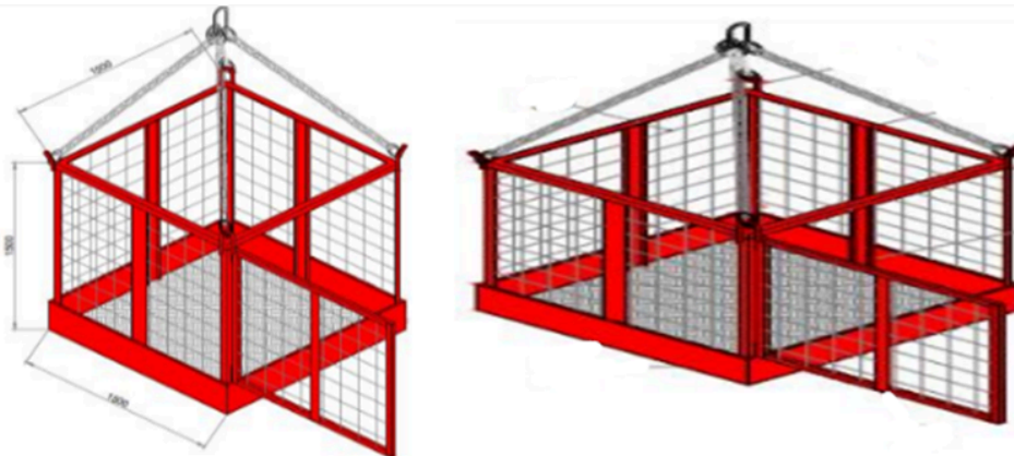
Figura 2. Modelo gaiola para transporte de materiais recicláveis.
