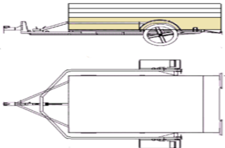
Figura 3 - carretinha basculante vedada.
