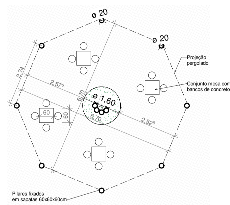
3 DETALHAMENTO PERGOLADO - BANCOS ESCALA 1:100
