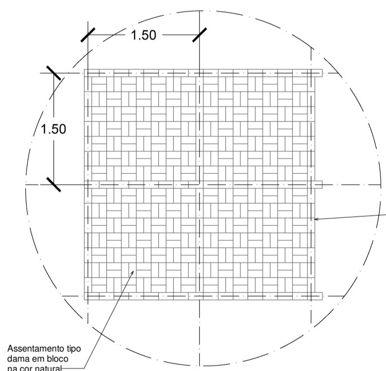
DETALHE PAGINAÇÃO 02 sem escala
