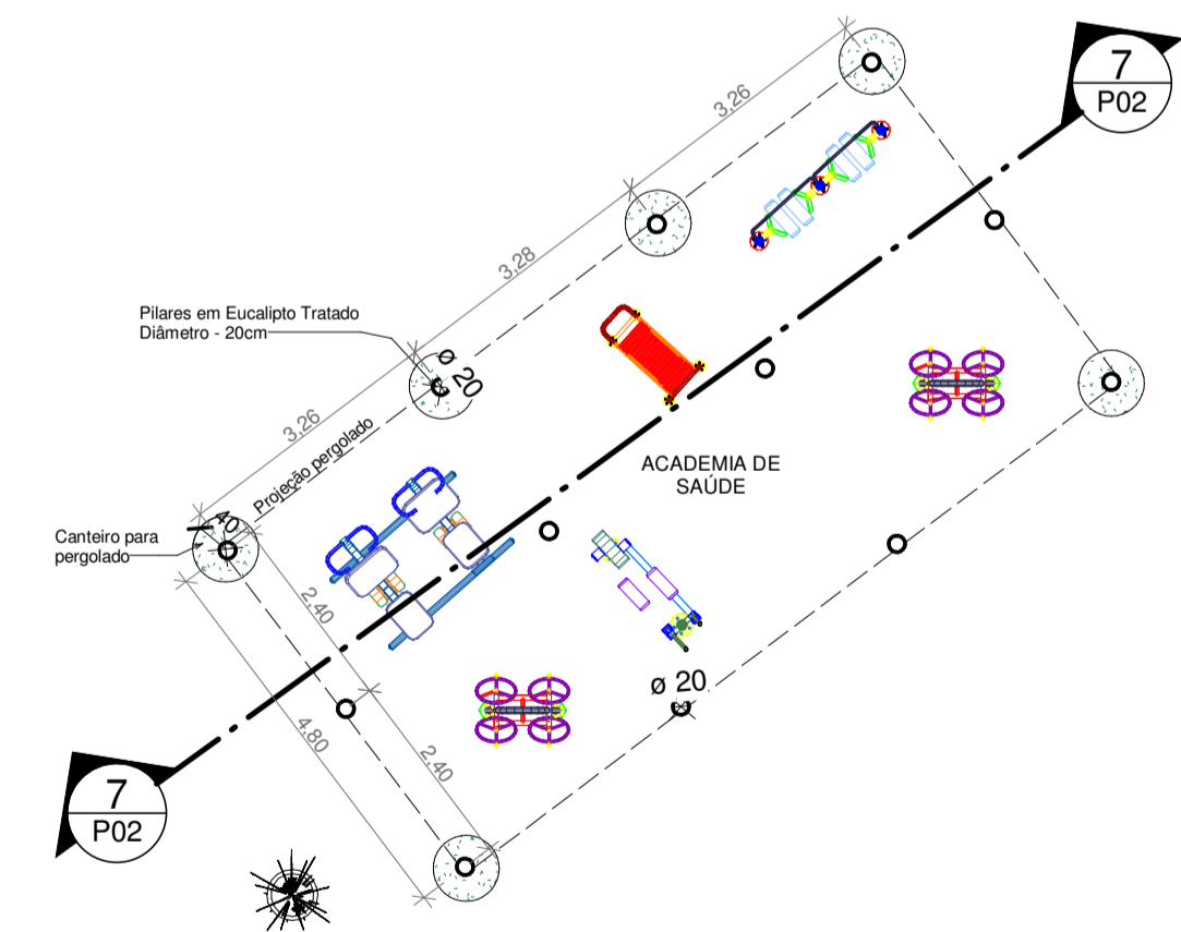
6 DETALHAMENTO PERGOLADO - ACADEMIA ESCALA 1:100
