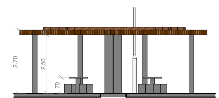
5 CORTE PERGOLADO - BANCOS ESCALA 1:100
