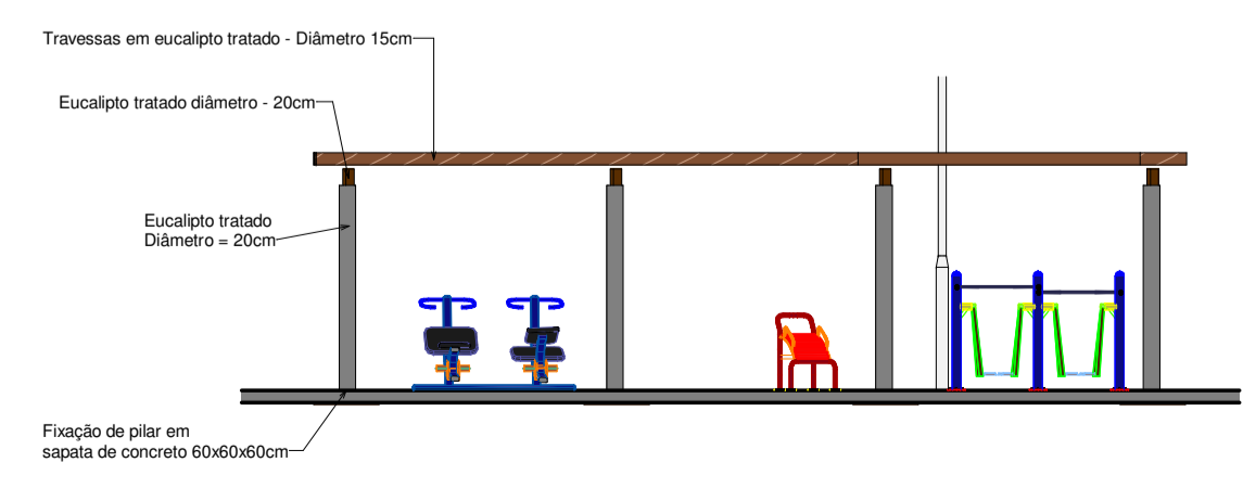
7 CORTE PERGOLADO - ACADEMIA ESCALA 1:100
