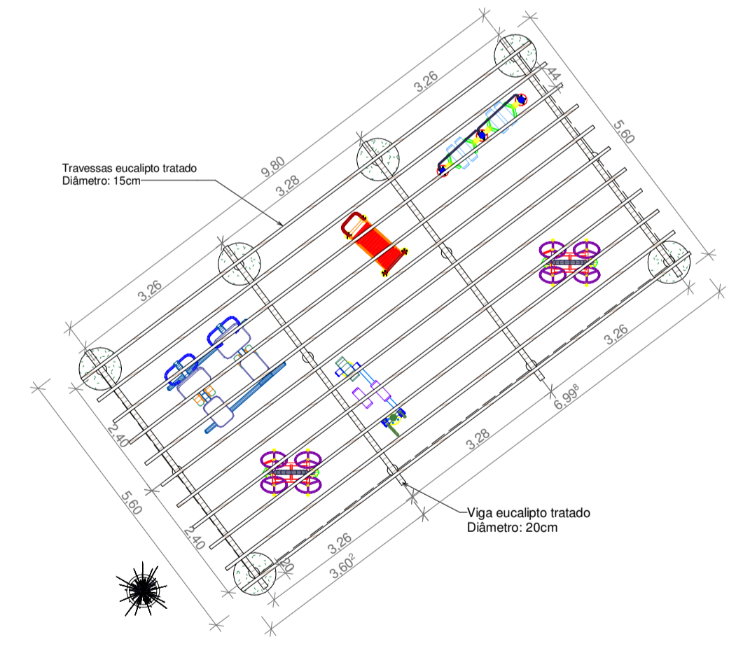
8 VISTA SUPERIOR PERGOLADO - ACADEMIA Copiar 1 ESCALA
