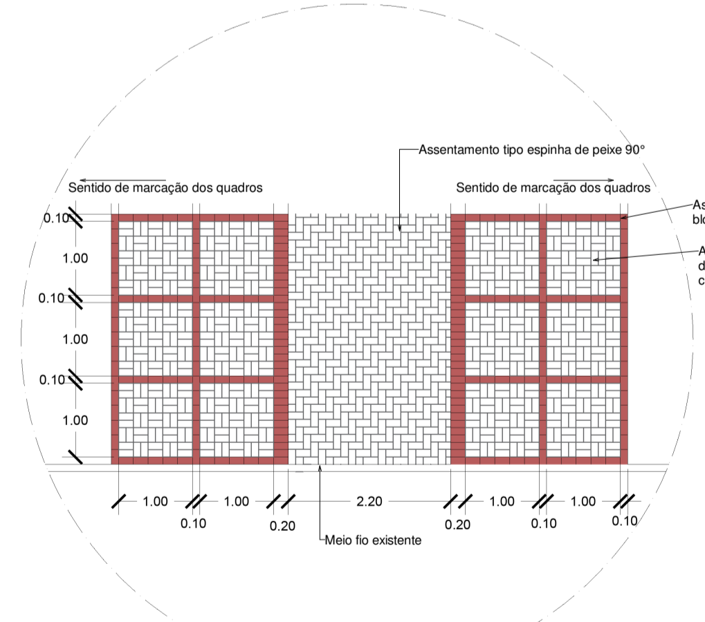
DETALHE PAGINAÇÃO 01 sem escala
