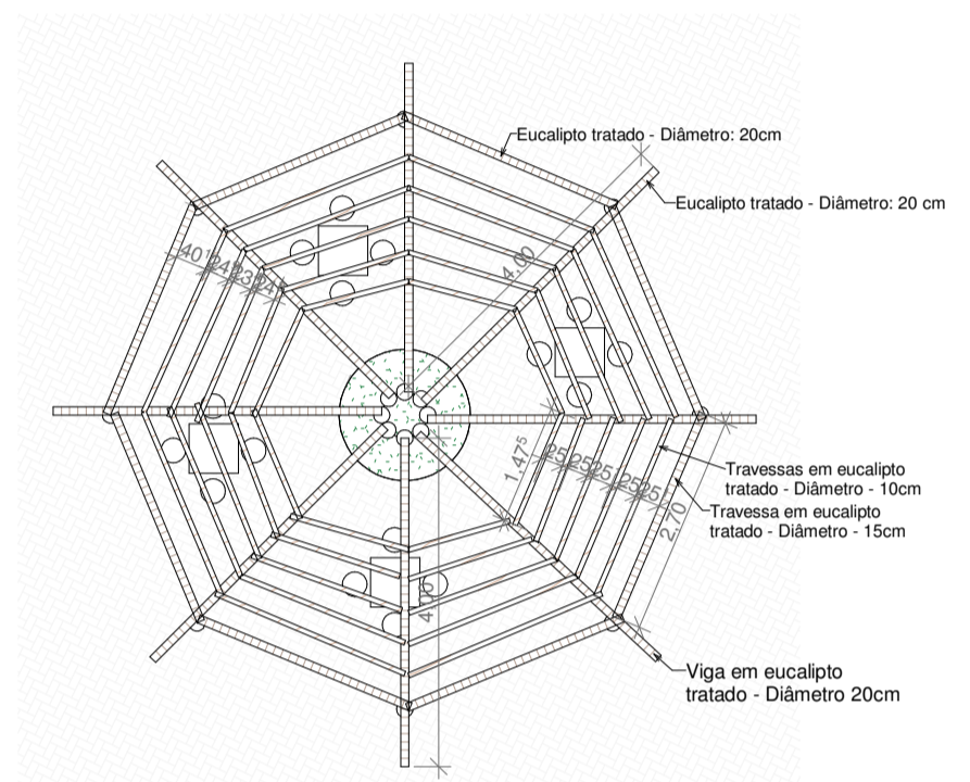
4 VISTA SUPERIOR PERGOLADO ESCALA
