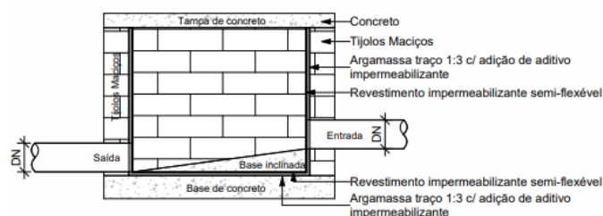
Detalhe típico caixa de injeção de esgoto
