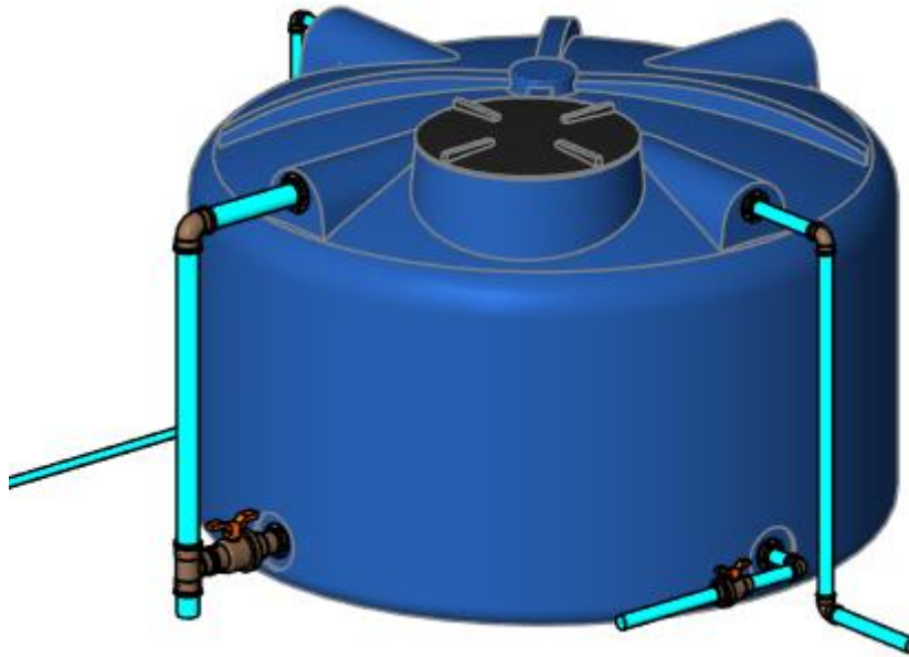
Tanque polietileno - 3.000 litros
