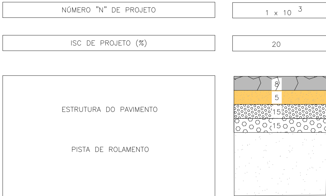
DIAGRAMA LINEAR DO PAVIMENTO
