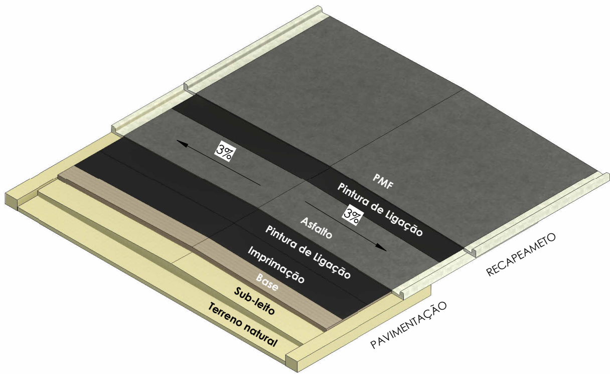
PERSPECTIVA DO RECAPEAMENTO - CAPA EM PMF ESC:
